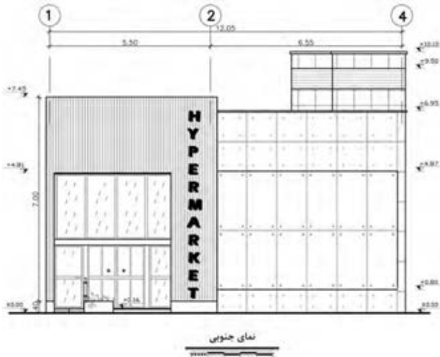
شکل ۵-۸۱- نقشه نما
