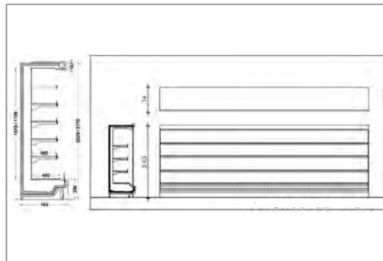
شکل ۵-۶۳- نقشه یخچال با ابعاد مورد نیاز
