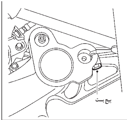
ب - محکم کردن بسیج بست‌ها شکل ۱۶۷-۳
