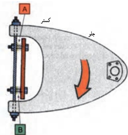
شکل ۲۲۲-۳- تغییر زاویه کمبر با واشرگذاری
