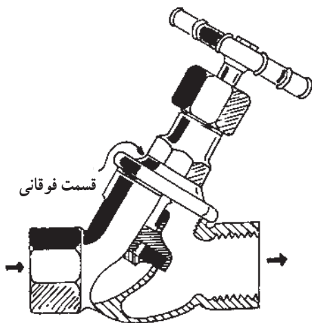
شکل ۲-۹۱- ب - شیر فلکه‌ی کف فلزی زاویه‌ای
