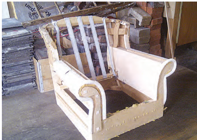
شکل ۷۰- اسکلت مبلی با اسفنج
