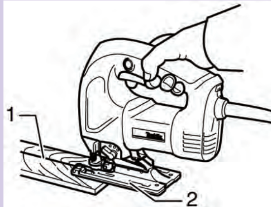
شکل ۴۱- برش مستقیم (۱- خط برش ۲- پایه)
