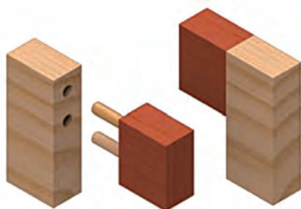
شکل ۲۶- اتصال دوبل
