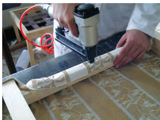
شکل ۶۲- ادامه منگنه زنی
