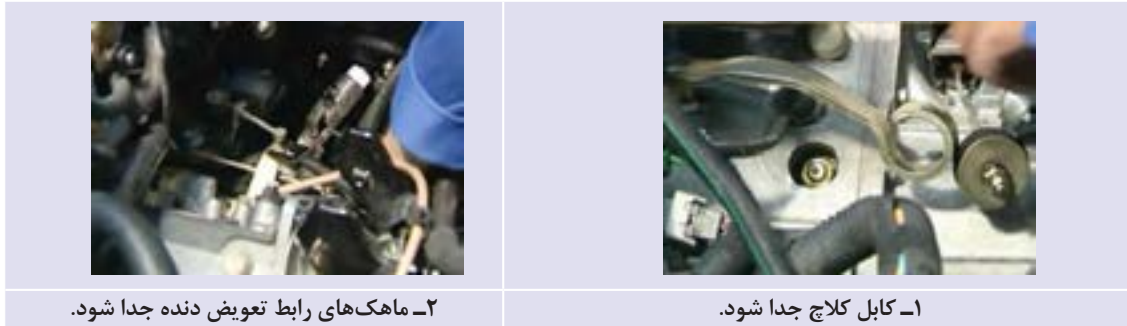
شکل ۹-۱۰- جدا نمودن اتصالات سیستم تعویض دنده
