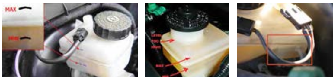
شکل ۵-۶- کنترل سطح مایع هیدرولیک ترمز
