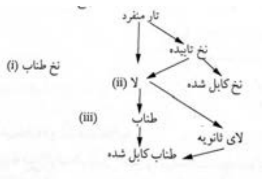
نمودار ۱ - ساختار کلی تولید انواع طناب‌های تابیده
