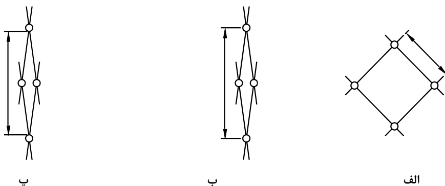
شکل ۴۳- نحوه اندازه گیری‌های مختلف چشمه تور، الف) طول ضلع چشمه - ب) طول چشمه، پ) اندازه حفره چشمه
