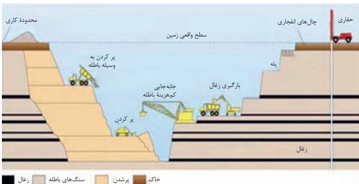
شکل ۳-۱-۳-۲-۱- نمای از یک معدن روباز زغال
