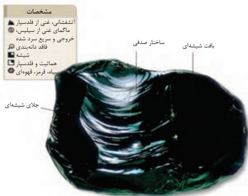
شکل ۲-۲۶- ابسیدین
