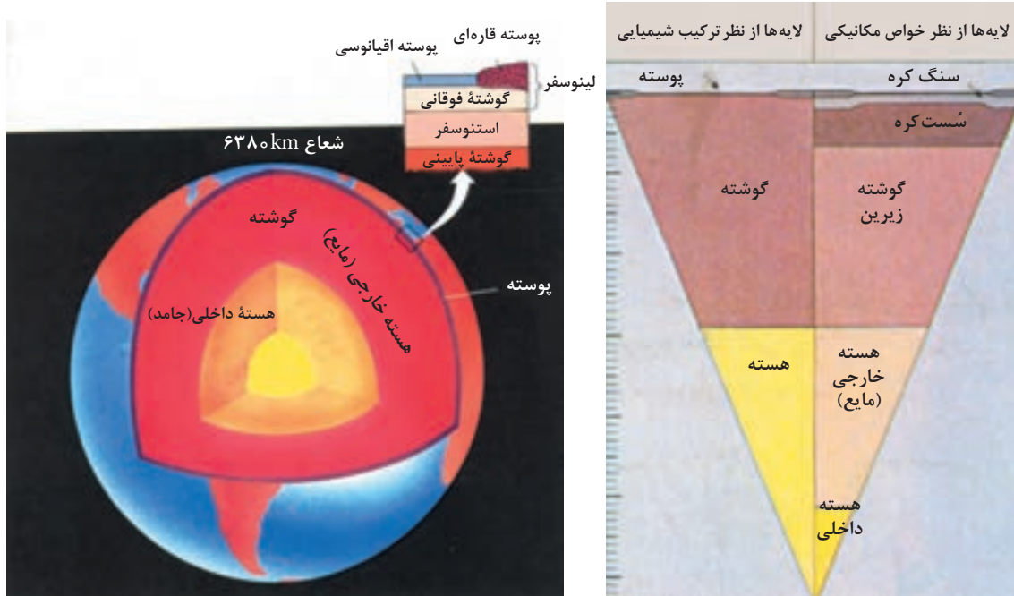
شکل ۲-۶- لایه‌های زمین (۴)
