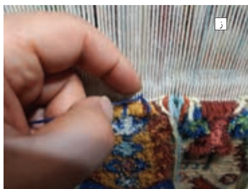
شکل ۱۱-۴- نحوه اجرای گره ترکی
