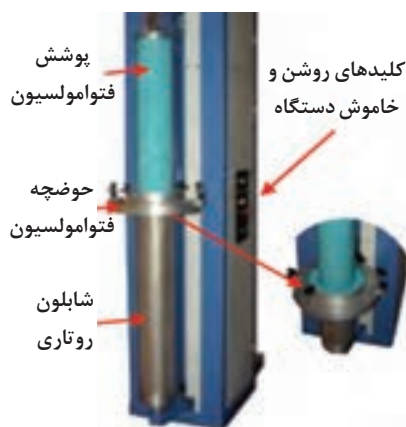
شکل ۲۳- ماشین لاک‌کشی روتاری
