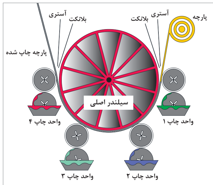
شکل ۱۵- نمای عملکردی ماشین چاپ غلتکی
