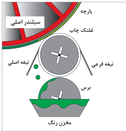
شکل ۱۶- اجزای مهم واحد چاپ گلته‌کی
