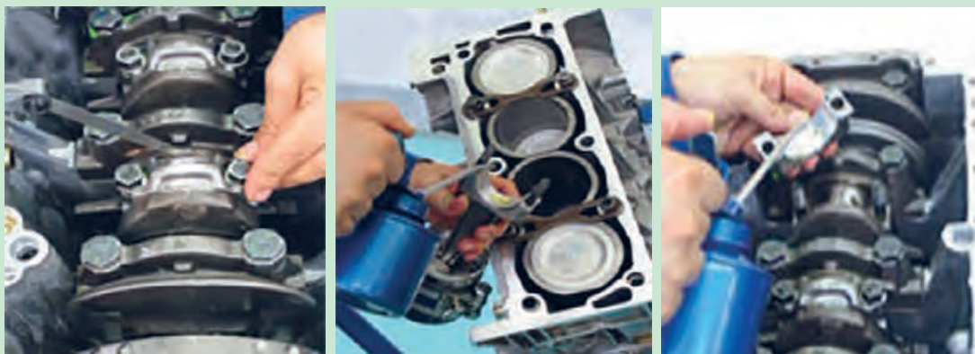
شکل ۱۰۲. کنترل لقی شاتون روی محور میل لنگ
