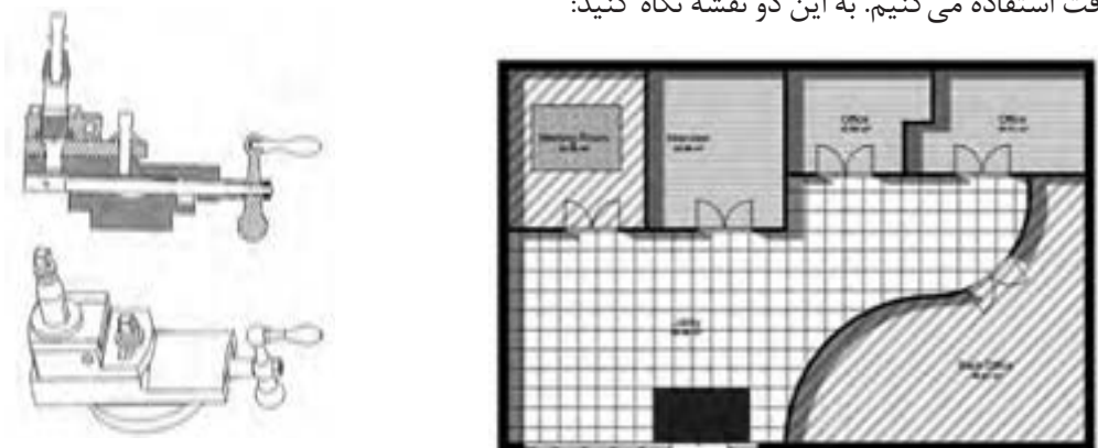
شکل ۱۳- در این نقشه برای تفکیک اتاق‌ها از هاشور استفاده شده است که در ضمن، معرف کفپوش آن‌ها نیز هست. شکل ۱۴- در این نقشه برای تفکیک قطعات در حالت برش خورده از هاشور استفاده شده است.
