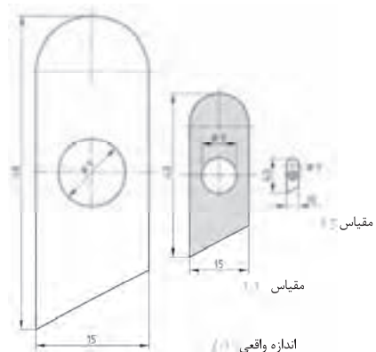
اندازه‌گذاری یک قطعه کار در مقیاس‌های مختلف
