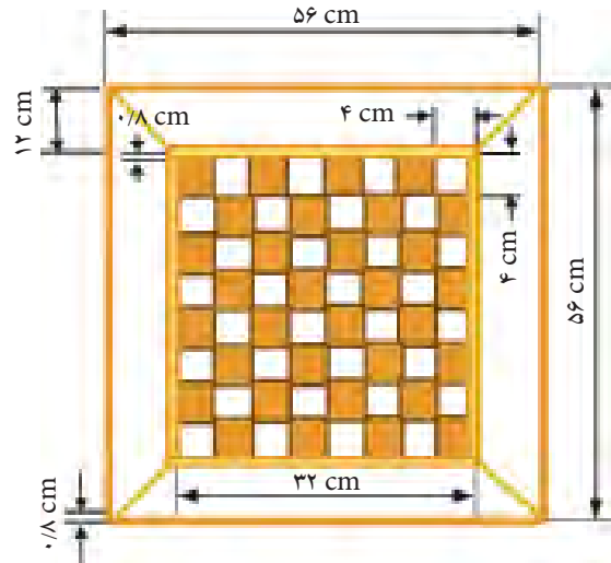
شکل ۱۶۴۰-۱۲. صفحه‌ی (رویه‌ی میز شطرنج).
