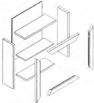
شکل ۸۲-۱۲- تصویر مجسم انفجاری جعبه‌ی کمک‌های اولیه.
