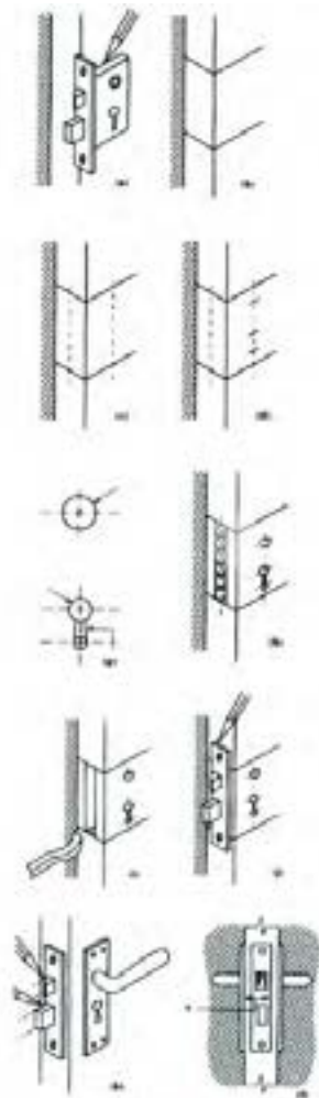
شکل ۱۱-۵۲ - مراحل مفصل جاسازی قفل.
