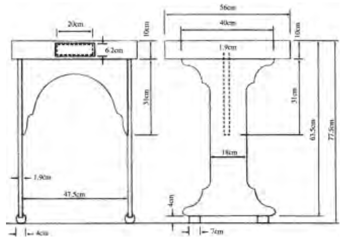
شکل ۱۶۵۹-۱۲. دو نمای اصلی میز شطرنج. ۵۶ cm
