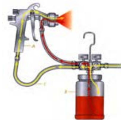
شکل ۴-۳۴- پیستوله با مخم کم.
