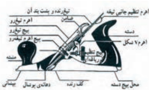
شکل ۲-۳- رنده‌ی دو تیغ فلزی
