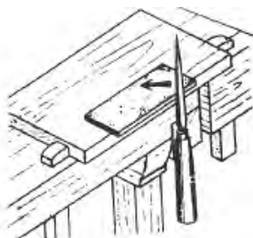
شکل ۹-۲- مصقل زدن به لبه‌ی لیسه با زاویه‌ی ۸۵ درجه.
