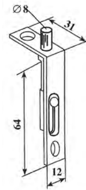
شکل ۱۰-۵۱- کشوی پشتی.
