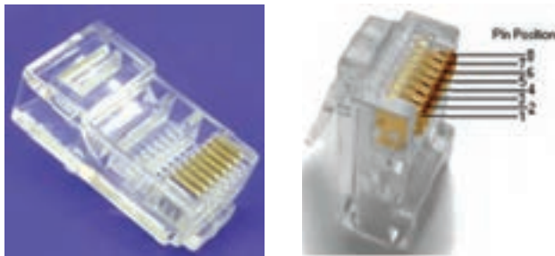
شکل ۴-۴۰- سوکت RJ45
