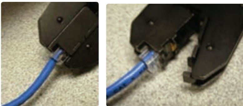
شکل ۴۷- پرس سوکت های کابل شبکه
