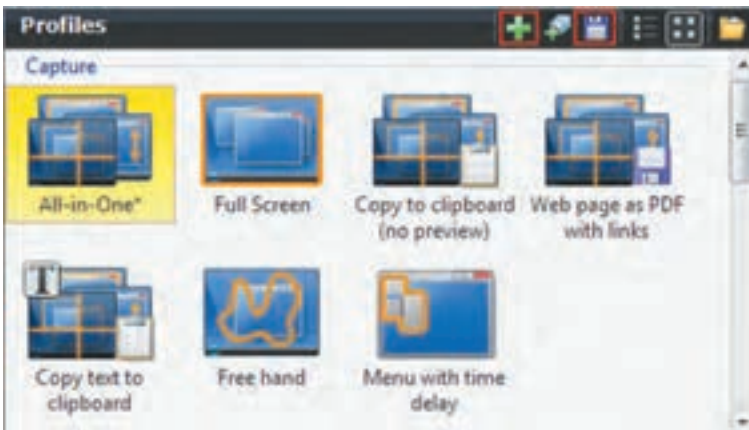
شکل ۲-۴۱- پنجره Profile
