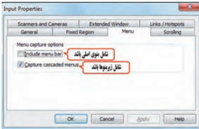
شکل ۱۴-۲. تنظیمات منو
