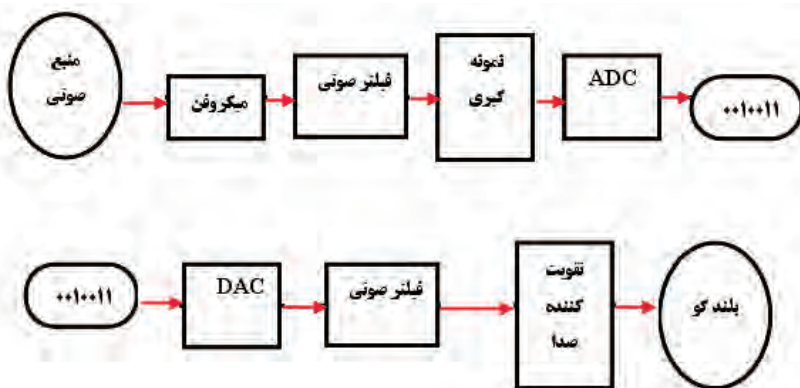
شکل ۵-۸-۱ عملکرد ADC و DAC
