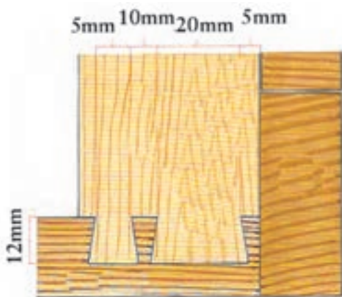
شکل ۵۷ - فایل اتصال دم‌چلچله در قید پایین پایه
