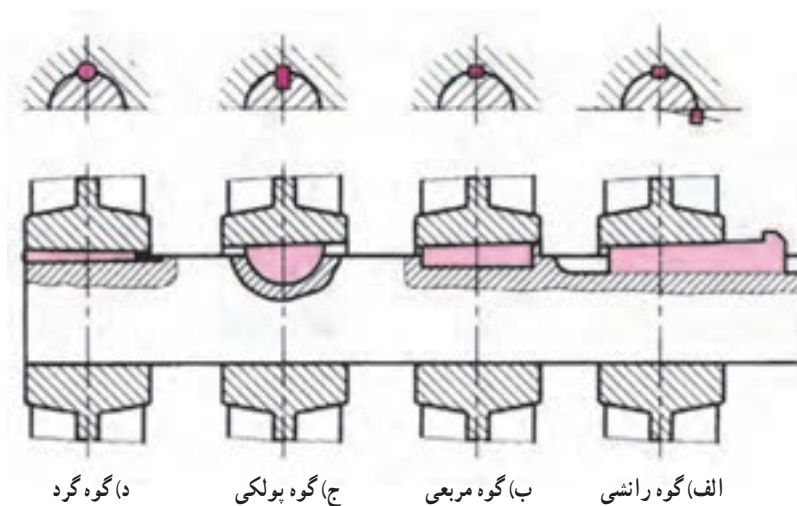
شکل ۲۲-۳- انواع گوه
