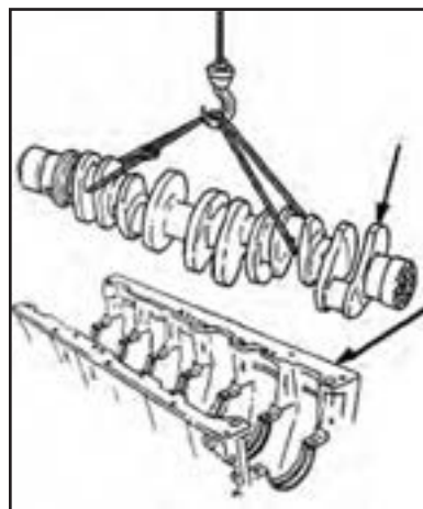
شکل ۱۵۵-۴- بلند کردن میل‌لنگ
