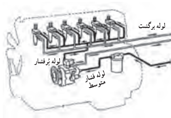
شکل ۳۳-۲- انواع لوله انتقال گازوئیل
