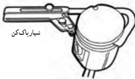
(الف) ابزار تمیزکننده شیپار رینگ‌ها
