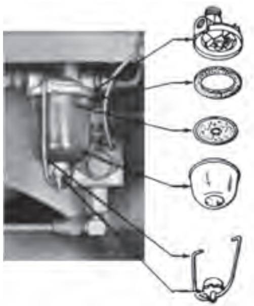
شکل ۱-۴- پیاله رسوب‌گیر
