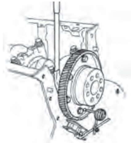
شکل ۱۷۹-۴- اندازه‌گیری لقی طولی میل‌لنگ با ساعت اندازه‌گیری
