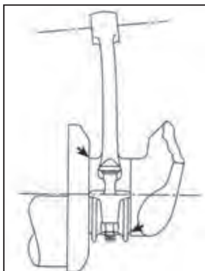
شکل ۱۱۰-۴- برخورد پیستون به سیلندر و شاتون به میل لنگ بر اثر خمیدگی بدنه شاتون
