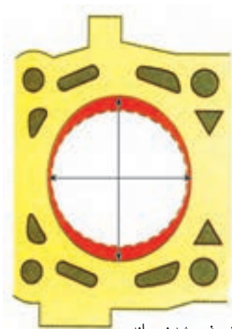
شکل ۱۴۹-۴- وضعیت بیضی شدن سیلندر
