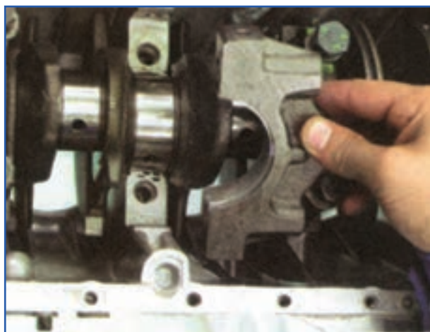
شکل ۱۸۹-۴ - جازدن کپه یاتاقان
