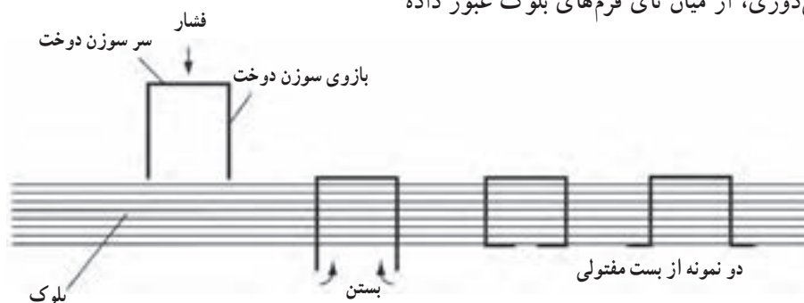
شکل ۵-۵- روش کار دوخت مفتولی و انواع بست مفتولی
