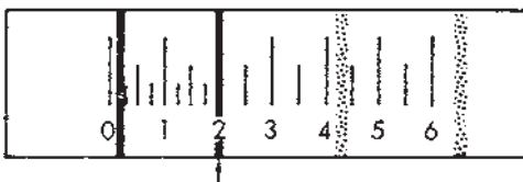
شکل ۹-۷- چگونه قرائت و اندازه‌گیری گاز متان به وسیله اینترفرومتر
