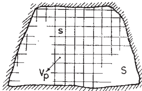
شکل ۲-۹- اندازه‌گیری سرعت هوا به وسیله‌ی سیم‌های نازک
