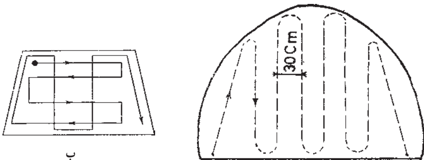
شکل ۲-۸- جهت حرکت دادن آنومتر در مقطع تونل برای اندازه‌گیری سرعت هوا
