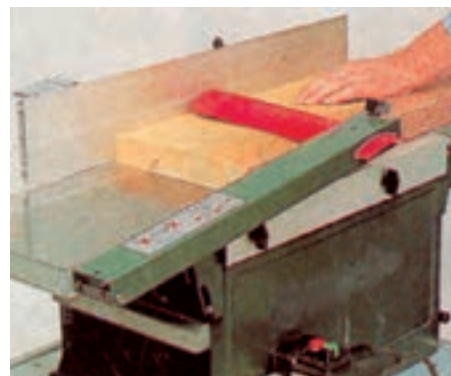
شکل ۴۱-۴- نحوه رندیدن روی سطح چوب با ماشین کوچک رنده
