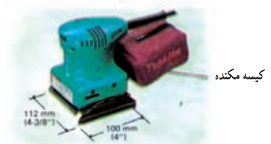
شکل ۱۲-۱۵ – سنباده لرزشی مکنده‌دار با قدرت ۱۶۰ وات
