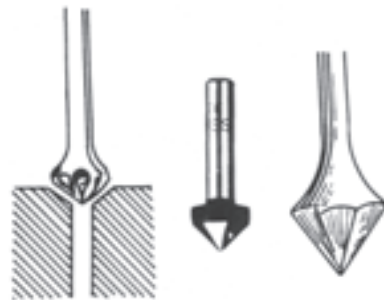
شکل ۹-۱۵/۱- مته خزینه
