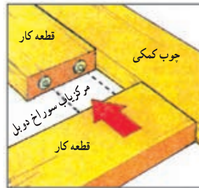
شکل ۱۰-۸- قطعه مرکز یاب سوراخ قطعه مجاور
