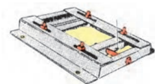
شکل ۲-۲۷ - پایه الکتروموتور با پیچ تنظیم پذیر
