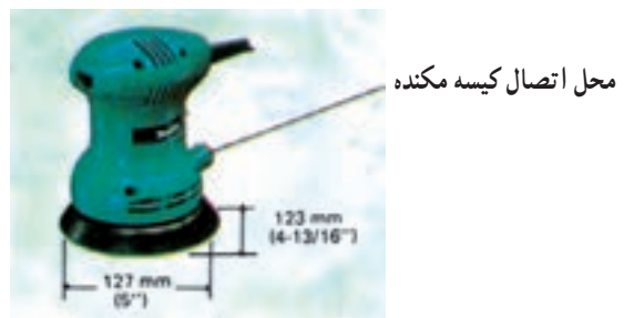
شکل ۱۲-۱۵ – سنباده لرزشی مکنده‌دار با قدرت ۱۶۰ وات
