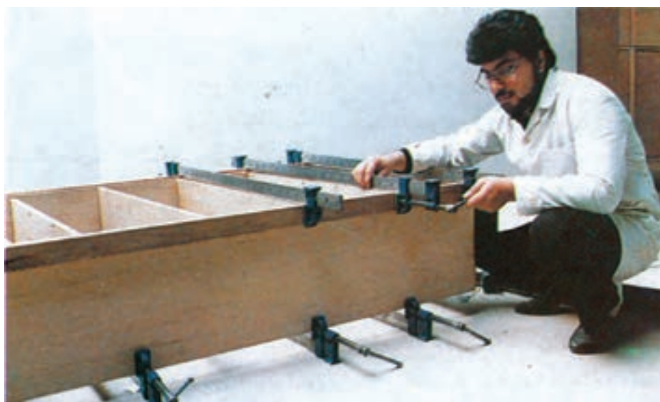
شکل ۲۲-۱۱- نحوه استقرار کتابخانه سر هم شده بین دهانه تنگ‌ها برای فشردن و چسباندن
