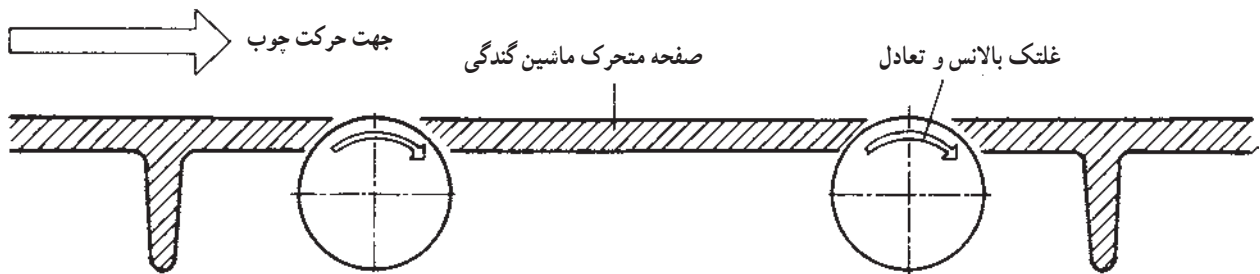
شکل ۴-۵۷- دو غلتک بالانس و تعادل صفحه ماشین گندگی برای کم کردن اصطکاک
