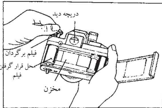
شکل ۴۴- بدنه دوربین
