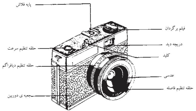
شکل ۴۲- دوربین عکاسی
