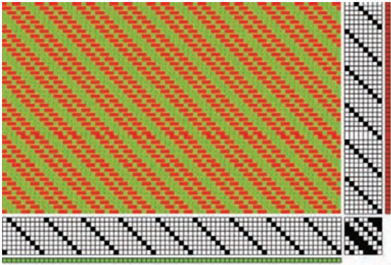
شکل ۲۳: طرح سرژه مرکب T \frac{201}{202} Z
