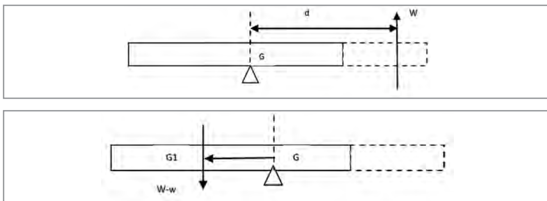
شکل ۲۲- جابه‌جایی مرکز ثقل تخته همگن پس از بریده شدن
