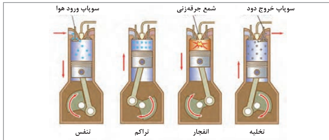
شکل ۱۷- موتور ۴ زمانه
