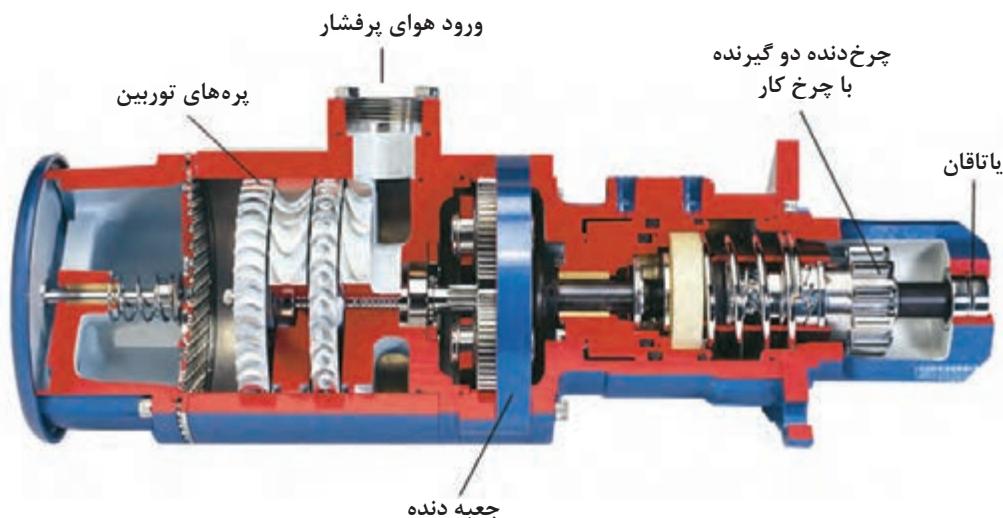
شکل ۴۰- موتور استارت هوایی
