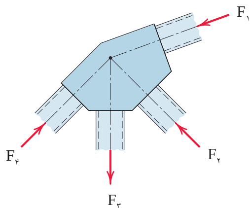
شکل ۷- نیروهای هم‌مرس وارده بر یک قطعه
