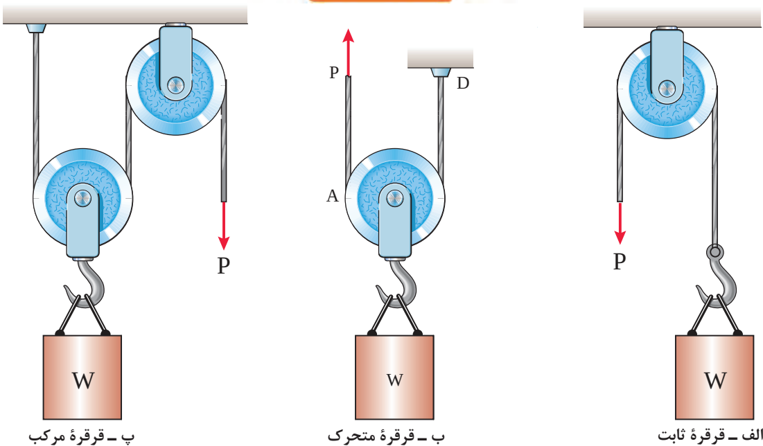
شکل ۲۳- انواع قرقره
