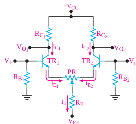
نقشه فنی تقویت کننده تفاضلی
