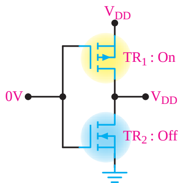
TR 1 وصل و TR 2 قطع
