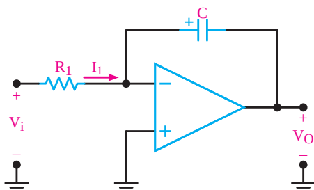
مدار انتگرال‌گیر
