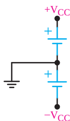
چگونگی ایجاد خط تغذیه متقارن
