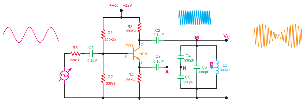
مدار مدولاتور ترانزیستوری AM
