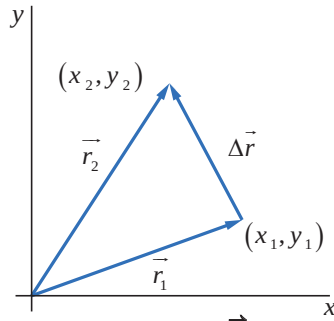
شکل ۲- بردار جابه‌جایی \Delta \vec{r} از تفاضل بردار موقعیت در لحظه اول و لحظه دوم به‌دست می‌آید.
