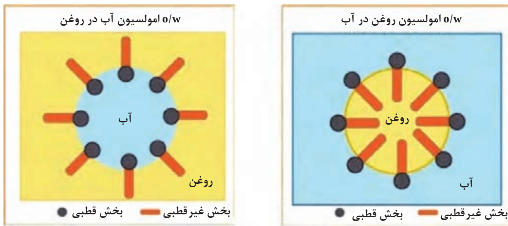
شکل ۹- شیوه تشکیل دو نمونه امولسیون o/w و w/o
