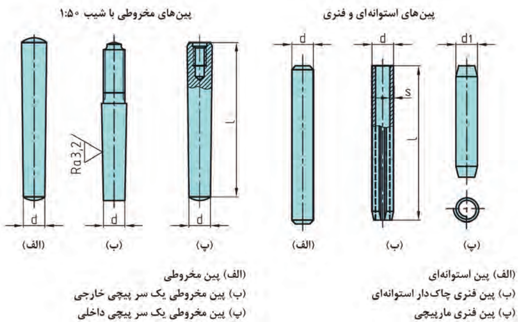
شکل ۹- پین ساده
