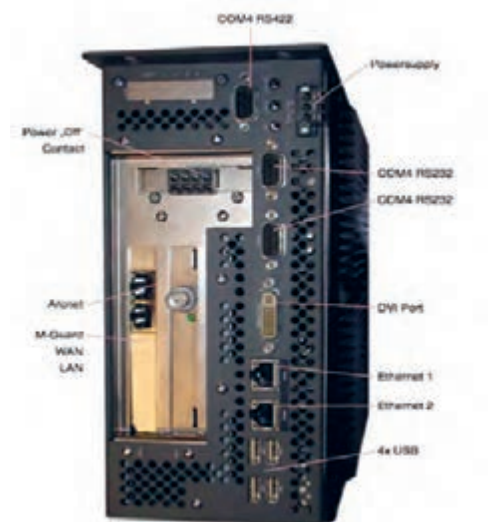
شکل ۲۳- یک نمونه کامپیوتر به همراه پورت‌های ارتباطی
