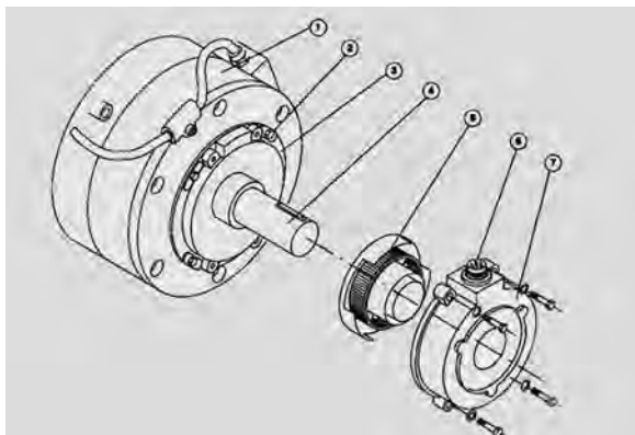
شکل ۲۳- مکانیزم کنترل حرکت (انکودر) موتور اصلی
