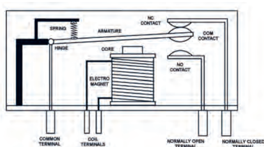
شکل ۲- ب) ساختمان داخلی رله
