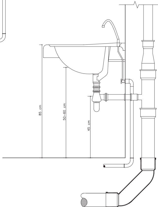
شکل ۲-۷۰ جزئیات روشویی
