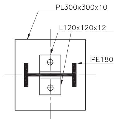
برش ۱-۱ (Sc: 1/10)
