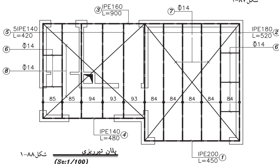
پلان تیرریزی (Sc:1/100)
