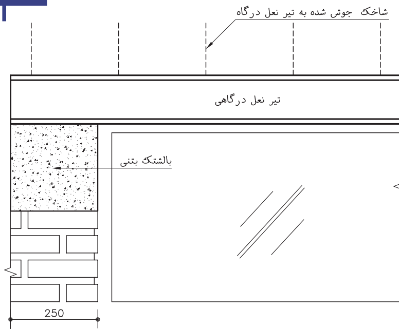
مشخصات نعل درگاه روی دیوار ۲۲ سانتی (Sc:1/10) شکل ۱-۷۱
