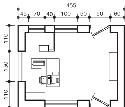
شکل ۱-۷۷ پلان اتاق نگرهانی
