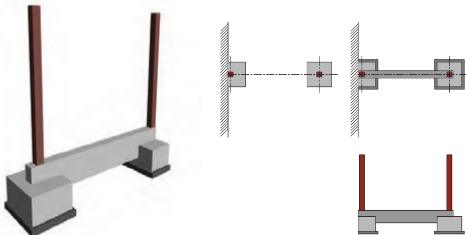
شکل ۱۴-۲- پی باسکولی
