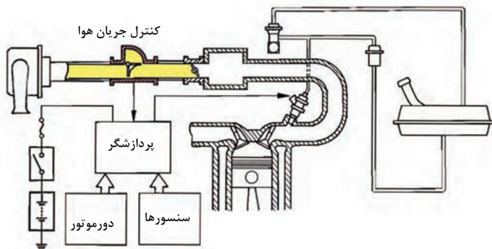
شکل ۳-۲- سیستم الکترونیکی پاشش بنزین نوع کنترل جریان هوا (L-EFI)
