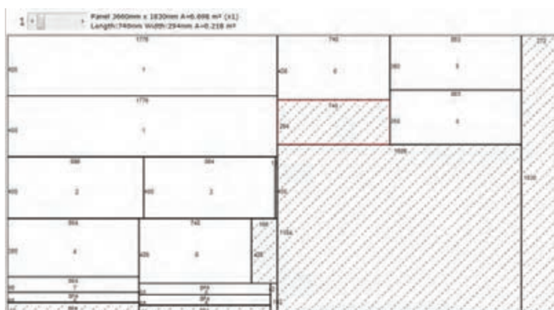
شکل ۲۳- ج - نقشه کات مستر زمانی که همه صفحات ۱۶ میلی‌متر را یک رنگ انتخاب نماییم.
