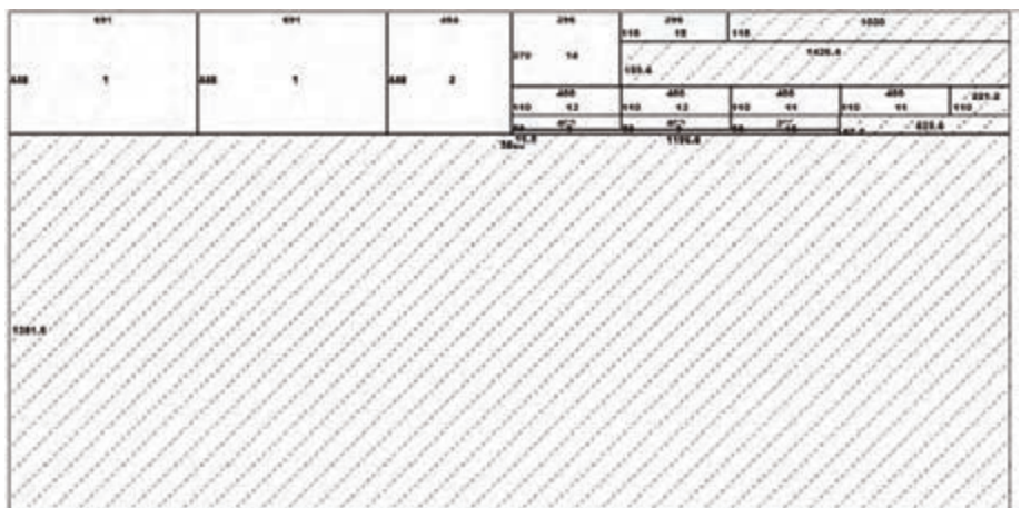
شکل ۲۸- نقشه چیدمان ورق رنگ طوسی ۱۶ میلی متر با ابعاد ۳۶۶×۱۸۳ سانتی متر
