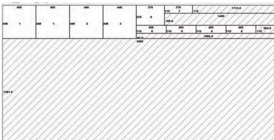
نقشه چیدمان ورق سفیدرنگ با ابعاد ۳۶۶×۱۸۳ سانتی متر
