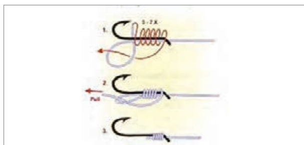
شکل ۲۴- دو نمونه گره برای بستن نخ مونوفیلament به قلاب ماهیگیری
