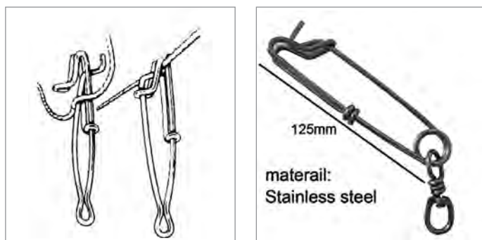
شکل ۲۹- گیره سنجاقی از جنس استینلس استیل و نحوه استفاده از آن برای اتصال به طناب اصلی
