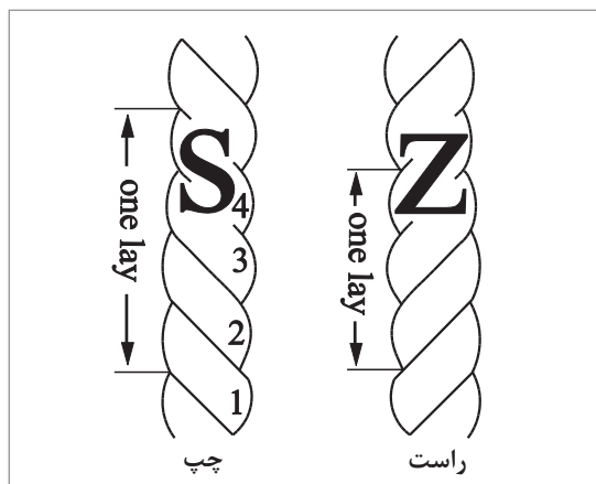
شکل ۱۴- انواع تاب (پیچش) در طناب‌های لیفی
