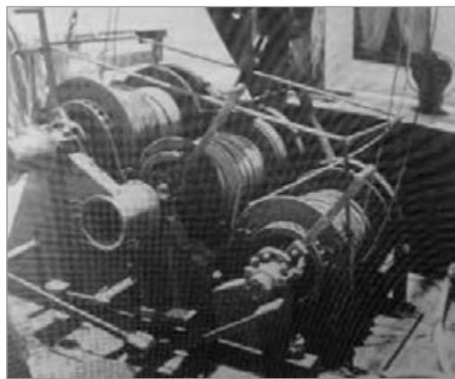
شکل ۵۴- نمونه‌ای از وینچ مورد استفاده در ترالرهای دو بازویی
