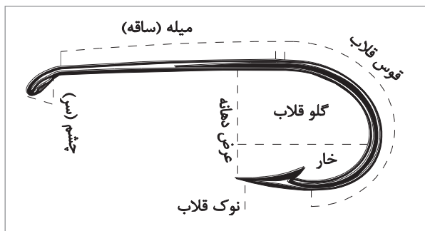
شکل ۲۲- قسمت‌های مختلف ساختمان یک قلاب ماهیگیری
