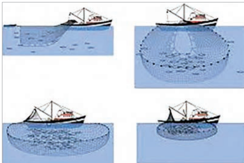
شکل ۶۱- مراحل مختلف عملیات صید با تور گردان پباله‌ای توسط کشتی پورس سینر
