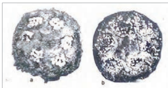
شکل ۱۳- مقطع عرضی دو نمونه طناب ترکیبی. a: طناب شش رشته با گرده بدون مغزه (هر گرده متشکل از ۱۱ سیم فولادی است)؛ b: طناب شش رشته با گرده‌های مغزه‌دار (هر گرده دارای ۲۸ سیم فولادی ظریف است)
