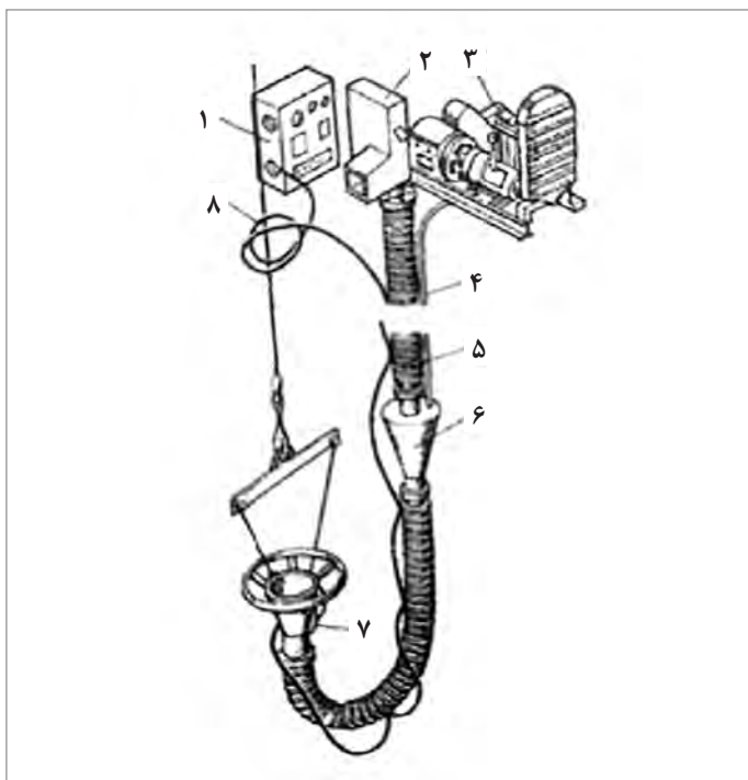
شکل ۴۵- ساختار پمپ و متعلقات آن
