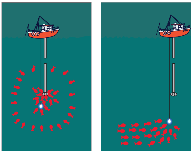
شکل ۴۴- مراحل مختلف صید کیلکا با پمپ، ۱- استقرار لوله متصل به پمپ و روشن نمودن لامپ در زیر آب و جلب ماهی‌ها به سمت آن، ۲- روشن نمودن پمپ و مکش ماهی‌های پیرامون چراغ
