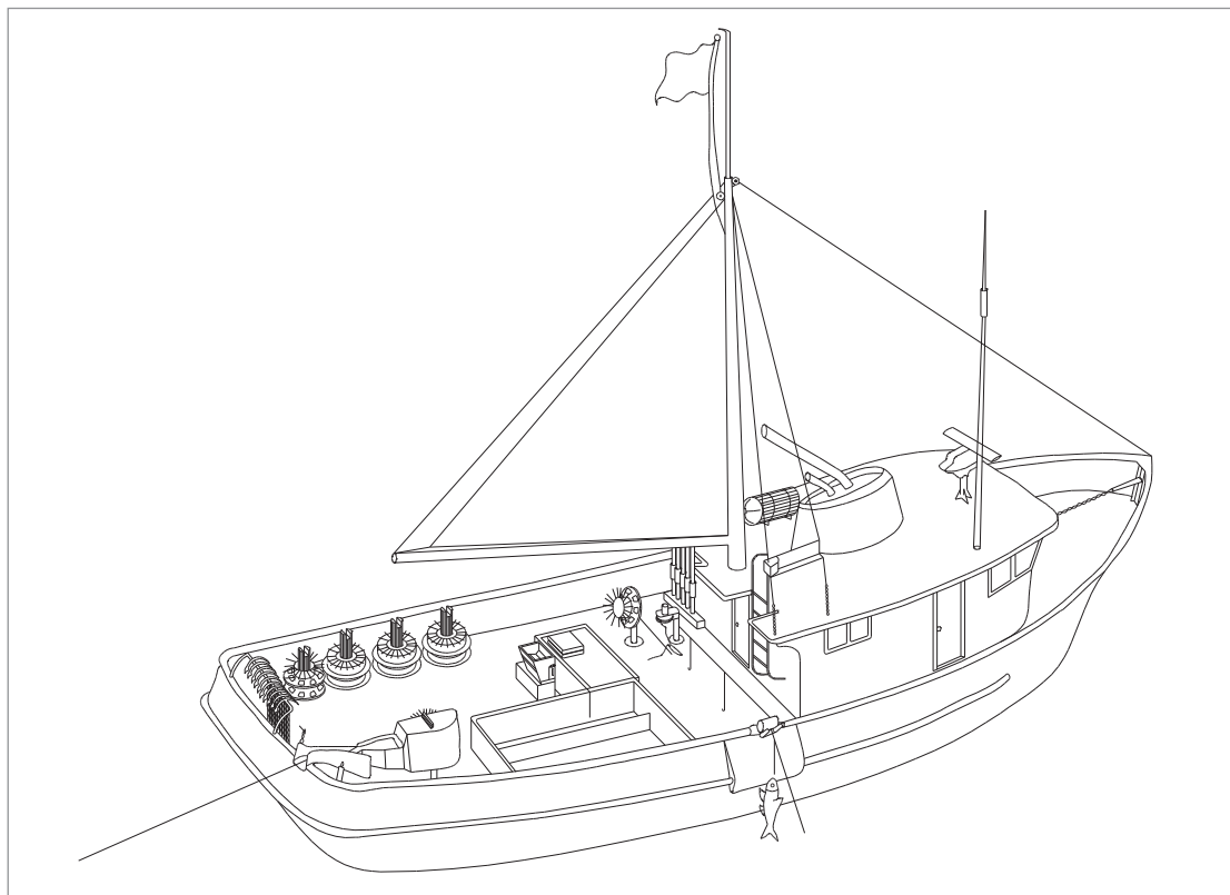
شکل ۲۳- کشتی ماهیگیری ویژه صید با رشته قلاب‌های طویل (لانگ لاینر)، ۱- ریل هدایت کننده طناب ۲- وینچ طناب ۳- قرقره طناب پیچ (قابل جدا شدن) ۴- محل نگهداری قرقره‌های طناب ۵- محل استقرار قرقره برای رها کردن طناب قلاب به دریا ۶- دستگاه طعمه خردکن ۷- طعمه زن اتوماتیک
