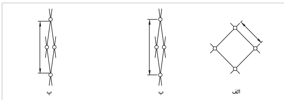
شکل ۴۳- نحوه اندازه‌گیری‌های مختلف چشمه تور، الف) طول ضلع چشمه، ب) طول چشمه، پ) اندازه حفره چشمه
