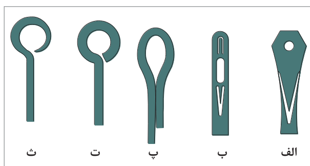
شکل ۲۳- انواع سر (چشم) در قلاب‌های ماهیگیری، الف) سر پهن، ب) سوزنی؛ پ و ت و ث) حلقوی
