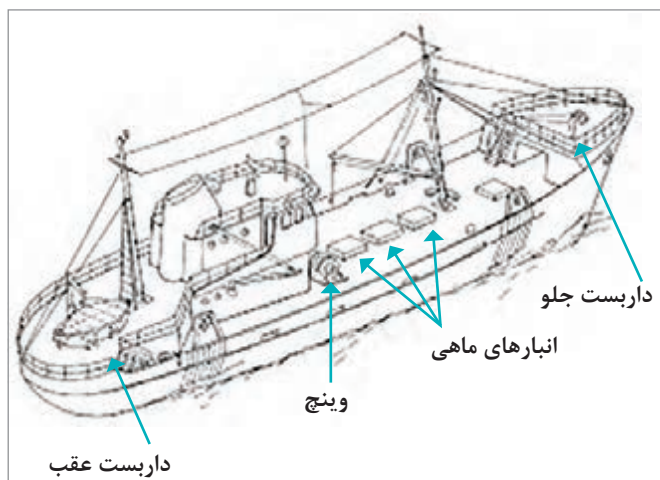
شکل ۴۷- یک نمونه کشتی ماهیگیری ترالر بغل کش
