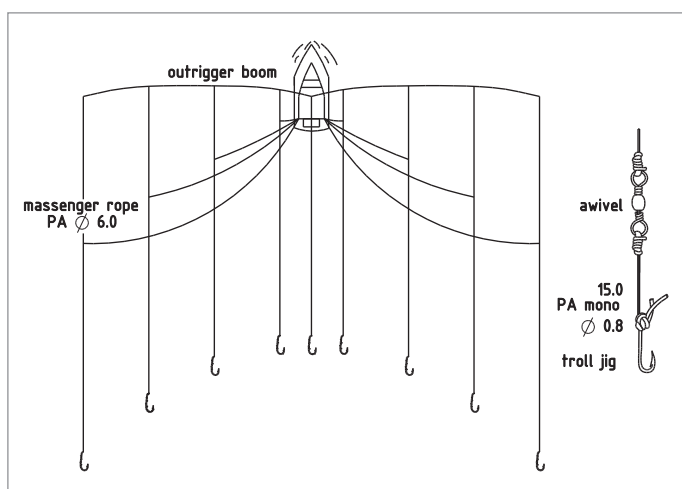
شکل ۳۱- نحوه چیدمان قلاب‌های کششی و مشخصات فنی مواد مورد استفاده در ساخت آنها
