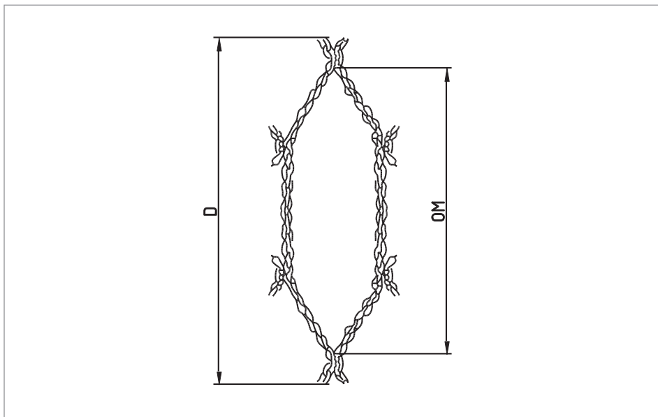
شکل ۳۸- چشمه شش ضلعی (الماسی شکل)، a = اندازه چشمه در حالت کشیده؛ OM = طول حفره چشمه در حالت کشیده (گره تا گره روبه‌رو)
