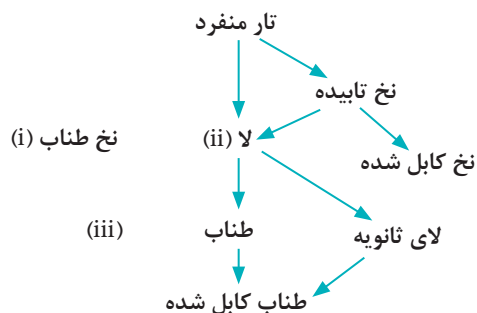
نمودار ۲- ساختار کلی تولید انواع طناب‌های تابیده
