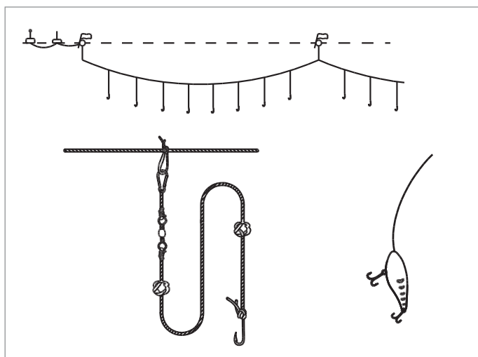
شکل ۳۲- ساختار کلی یک رشته قلاب طویل و اجزای آن
