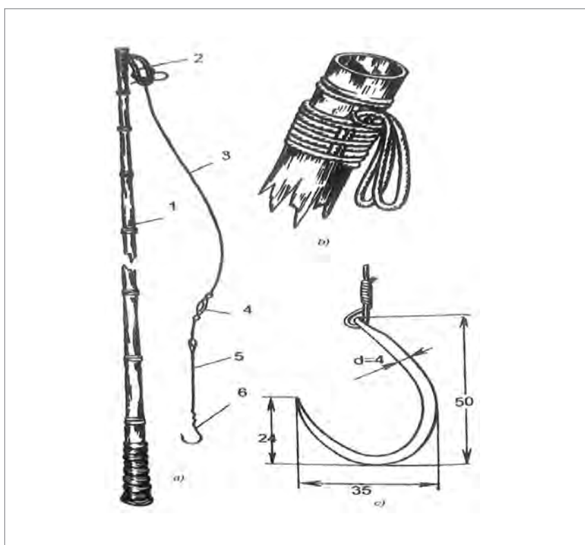
شکل ۳۶- قلاب و دسته از جنس خیزران و مشخصات و اجزای مختلف آن: (۱- خیزران، ۲- حلقه اتصال نخ، ۳- نخ اصلی، ۴- هرزگرد، ۵- نخ (سیم) ثانویه، ۶- قلاب)
