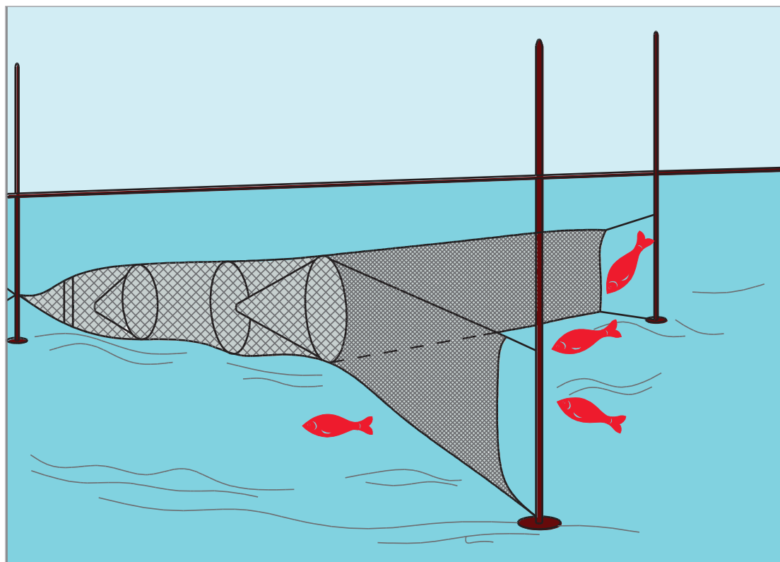
شکل ۱۵- تله تونلی ثابت با بال‌های جانبی
