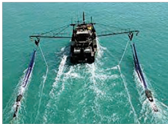
شکل ۵۳- تصویر عملیات توراندازی توسط یک کشتی ماهیگیری ترالر دو بازویی از نمای پشت
