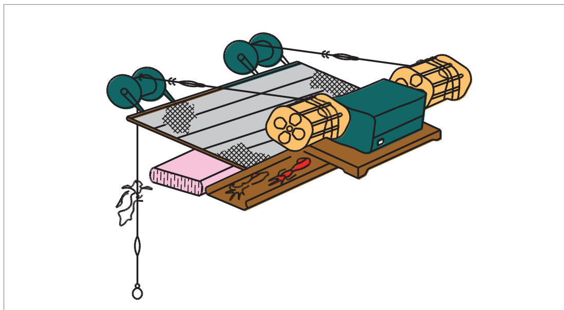
شکل ۳۱- دستگاه اتوماتیک صید اسکوئید به روش جیگینگ
