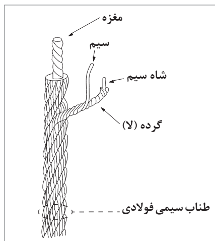
شکل ۱۵- ساختار کلی یک طناب سیمی
