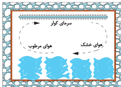
شکل ۲۷- جریان هوا در داخل سردخانه
