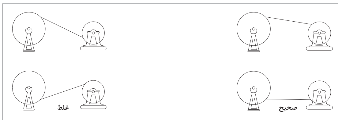
شکل ۲۰- اصول پیچاندن طناب‌های سیمی از روی یک قرقه به قرقه دیگر
