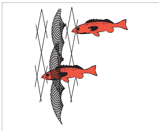
شکل ۳۷- ساختار یک تور سه لایه (ترامل نت) و موقعیت بافته‌های توری نسبت به یکدیگر
