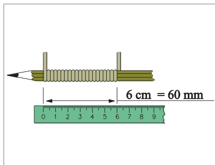
شکل ۶- نحوه محاسبه قطر نخ با استفاده از خط کش
