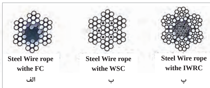
شکل ۱۶- انواع مغزه و نحوه استقرار آنها در طناب‌های سیمی
