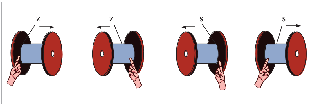
شکل ۲۱- نحوه جمع کردن وایر بر روی قرقره یا بشکه وینچ با توجه به جهت تاب آن
