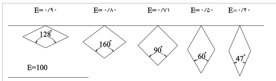
شکل ۴۴- وضعیت چشمه‌های تور در ضرایب مختلف آویختگی
