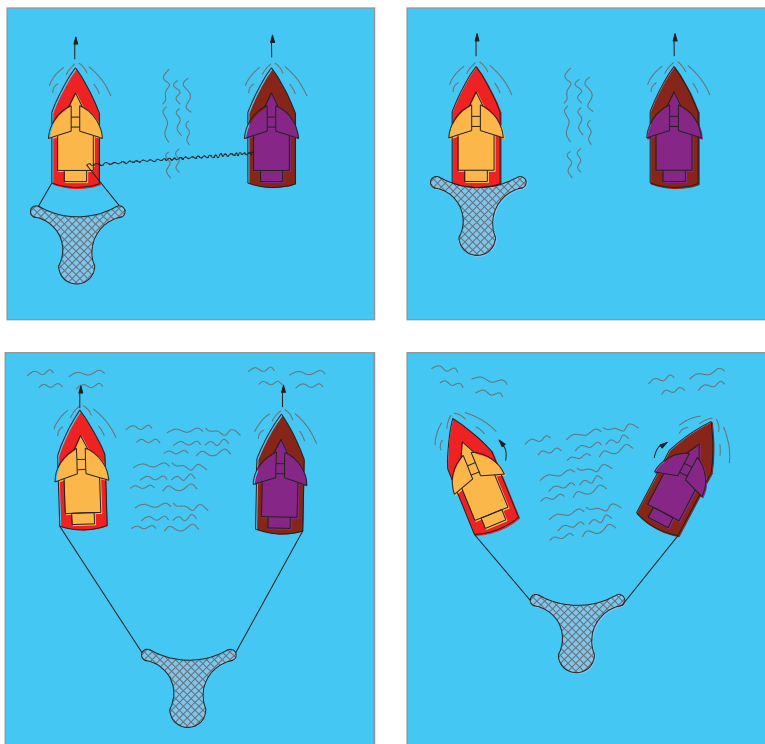
شکل ۴۹- مراحل مختلف عملیات ماهیگیری با ترالهای زوجی
