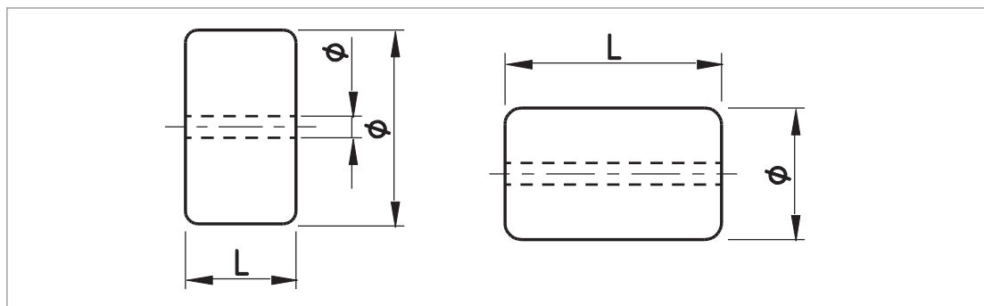
شکل ۴۷- نحوه اندازه‌گیری ابعاد و مشخصات فنی دو نمونه کرف استوانه‌ای
