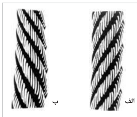
شکل ۱۷- انواع تاب در طناب‌های سیمی، (الف) راست تاب Z، (ب) چپ تاب S
