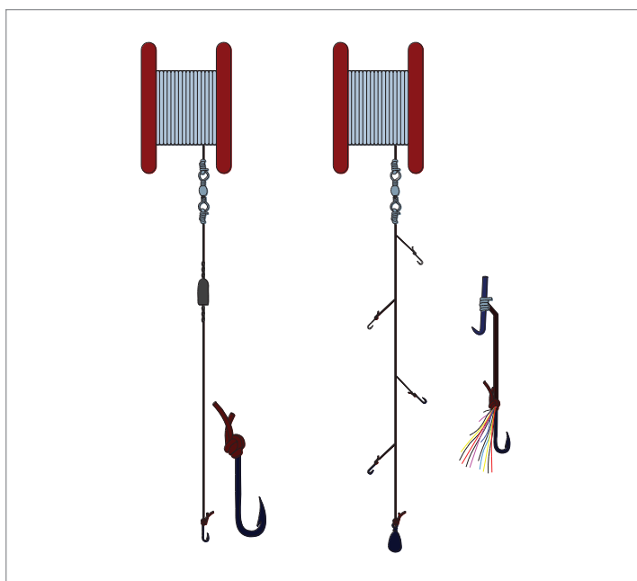
شکل ۳۰- دو نمونه قلاب دستی با شرح جزییات فنی مصالح استفاده شده در آنها الف) قلاب دستی با قلاب‌های متعدد، ب) قلاب دستی با قلاب منفرد
