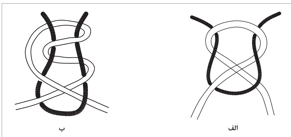
شکل ۳۹- دو نمونه گره مرسوم در بافت تورهای گره‌دار: الف) گره خفت کتابی ساده (Weaver's knot)، ب) گره خفت کتابی مضاعف Double weaver's knot
