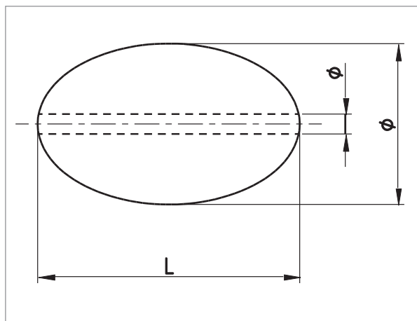
شکل ۴۵- نحوه اندازه‌گیری ابعاد و مشخصات فنی یک کرف بیضوی
