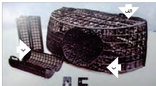
شکل ۱۳- اجزای یک قفس ویژه صید شاه میگو (لایستر): (الف بدنه قفس؛ ب قفل یا بست؛ پ طعمه دان.
