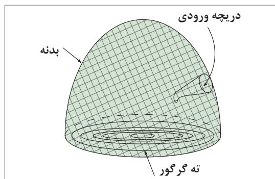
شکل ۹- ساختمان یک گرگور سیمی و اجزای سه‌گانه آن
