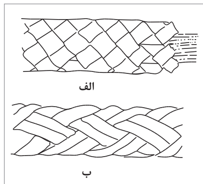
شکل ۴- ساختار نخ‌های بافته شده، (الف) گیس باف، (ب) لوله‌ای با مغزه
