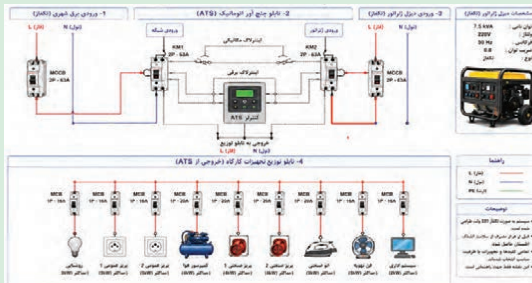
شکل ۲۶- نقشه شماتیک تابلو چنج آور اتوماتیک (ATS) - سیستم تک فاز
