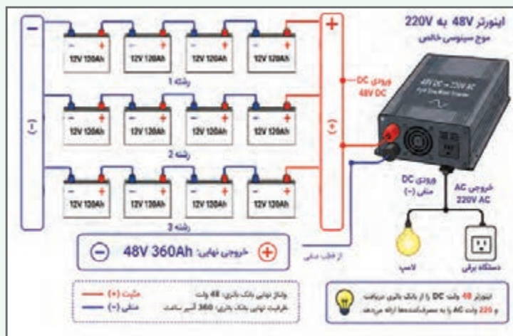
شکل ۶- اتصال اینورتر به باتری
