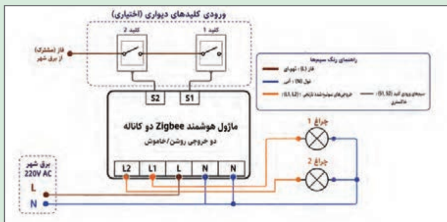
شکل ۴۳- اتصال تجهیزات روشنایی در پروتکل Zigbee
