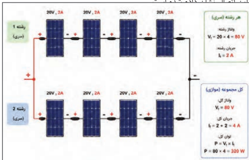
شکل ۲۷- اتصال سری - موازی دو رشته پنل ۴ تایی
