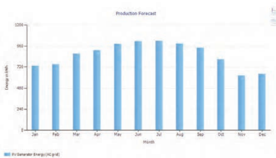
شکل ۶۱- نمودار پیش بینی تولید
