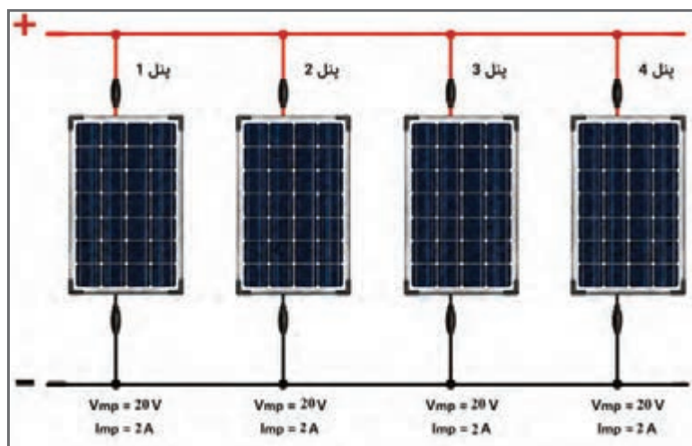
شکل ۲۵- اتصال موازی چهار پنل یکسان
