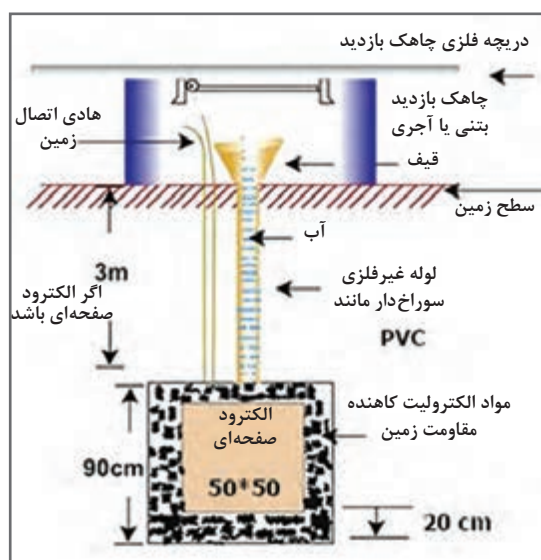
شکل ۲۷- الکتروود صفحه‌ای
