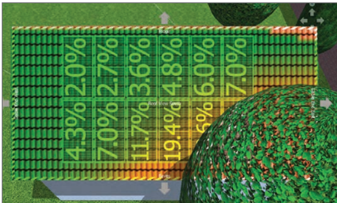
شکل ۵۶- اثر سایه بر روی پنل‌ها
