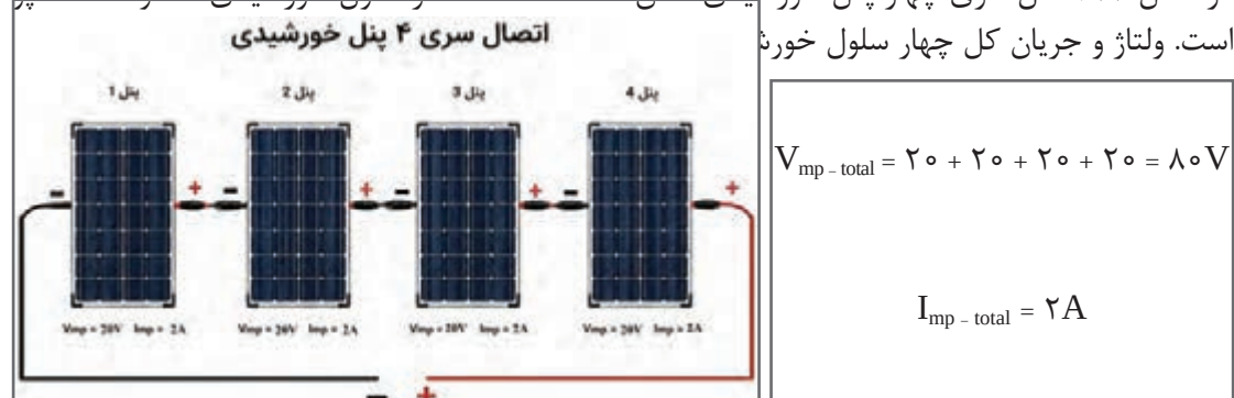
شکل ۲۳- اتصال سری چهار پنل یکسان
