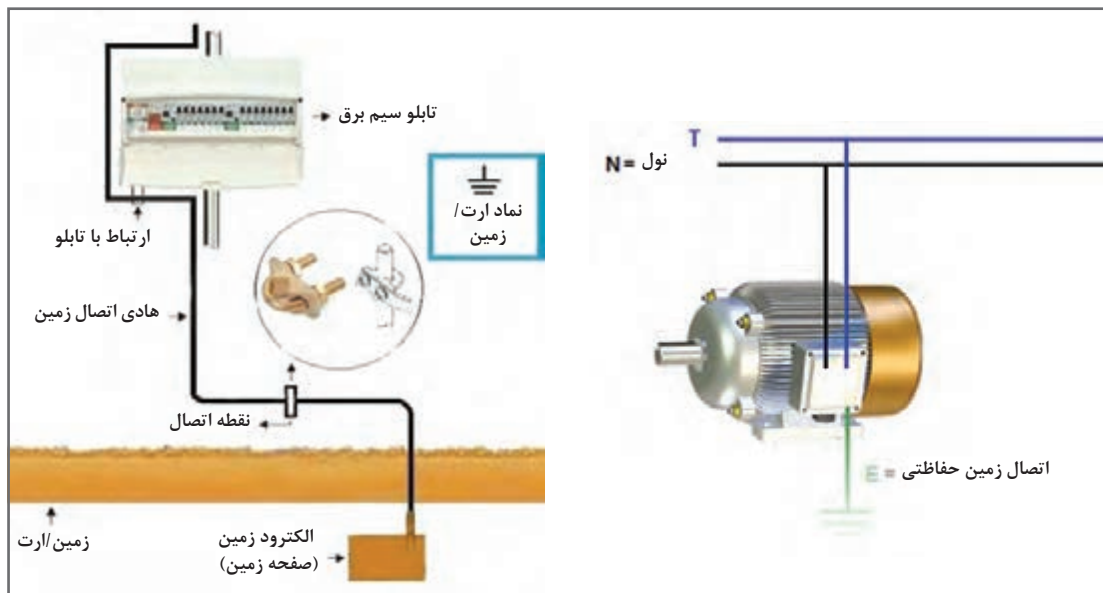
شکل ۲۴- سیستم اتصال زمین
