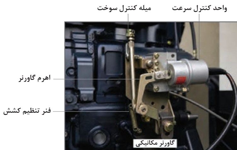
شکل ۳- یک نمونه از گاورنر مکانیکی به همراه جزئیات
