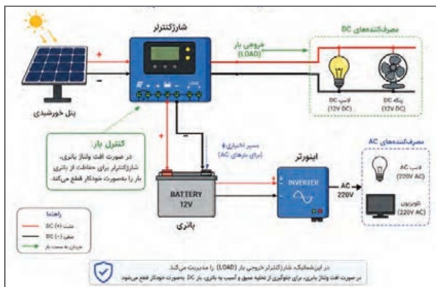
شکل ۲- نمایش سامانه مستقل از شبکه
