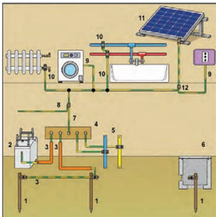
شکل ۱۷- سیستم هم‌بندی
