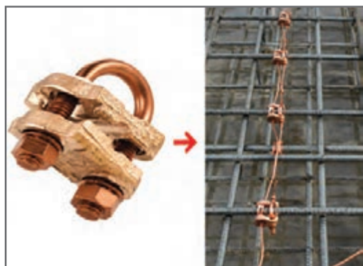
شکل ۱۹- بست U-type
