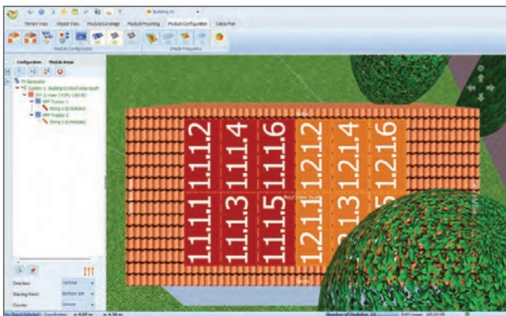
شکل ۵۸- آرایش پنل‌ها و جداسازی هر رشته با رنگ و کد مشخص
