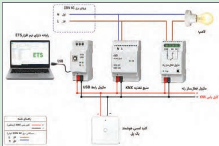
شکل ۹- اتصال کلید هوشمند لمسی به عملگر برای کنترل یک لامپ
