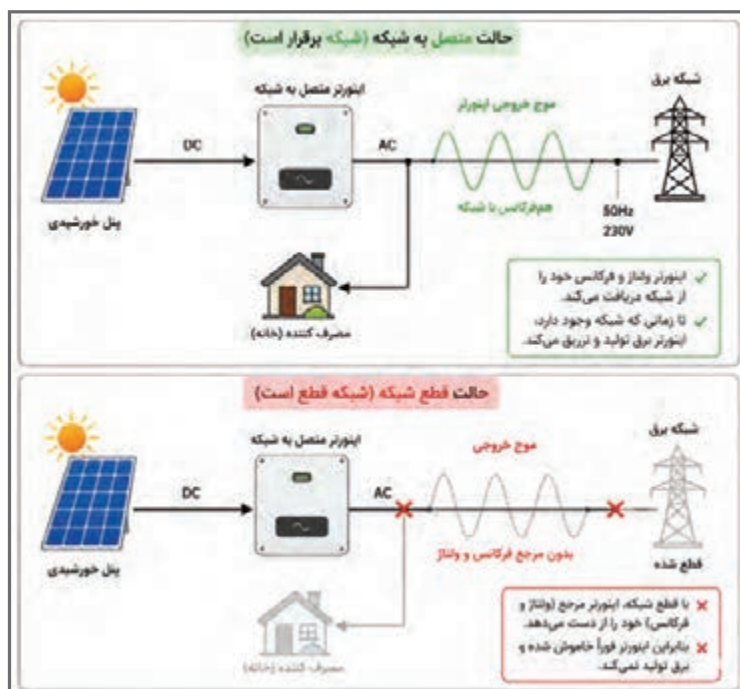
شکل ۳۷- عملکرد تنظیم ولتاژ و فرکانس در دو حالت متصل به شبکه و قطع شبکه
