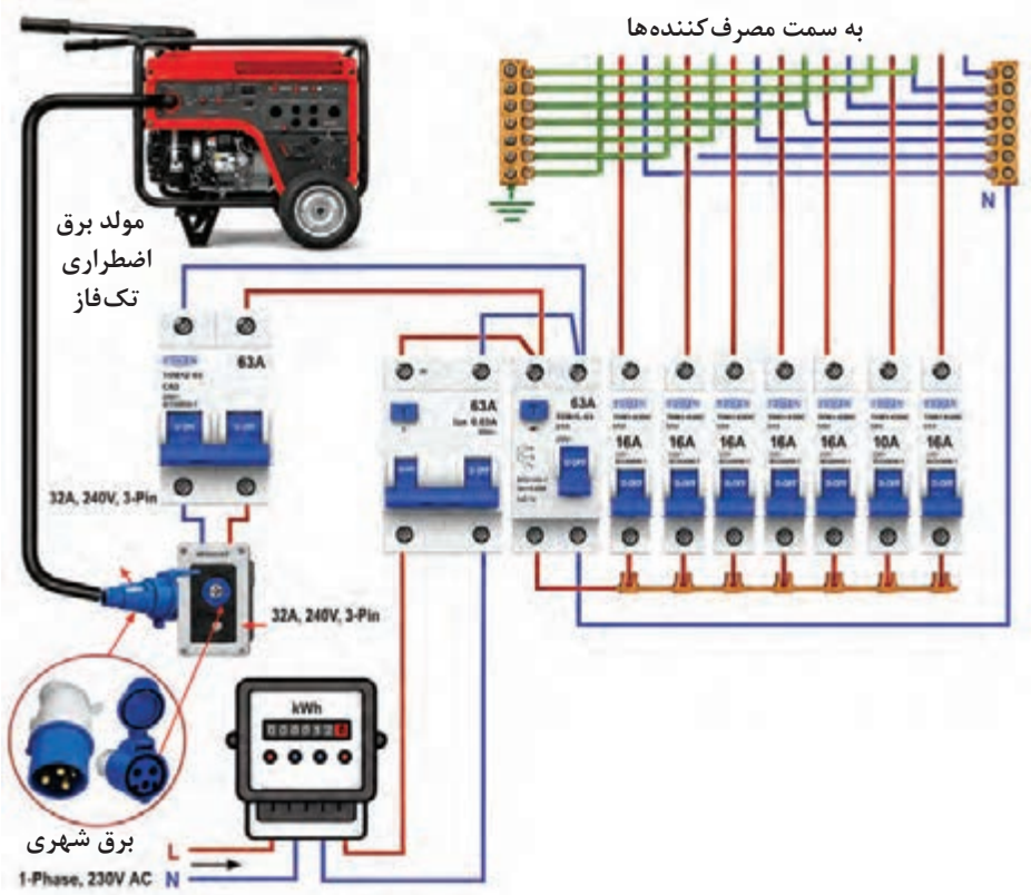
شکل ۱۸- نحوه اتصال مولد و شبکه سراسری به بار با دو کلید مجزا (بدون کلید چنج آور)
