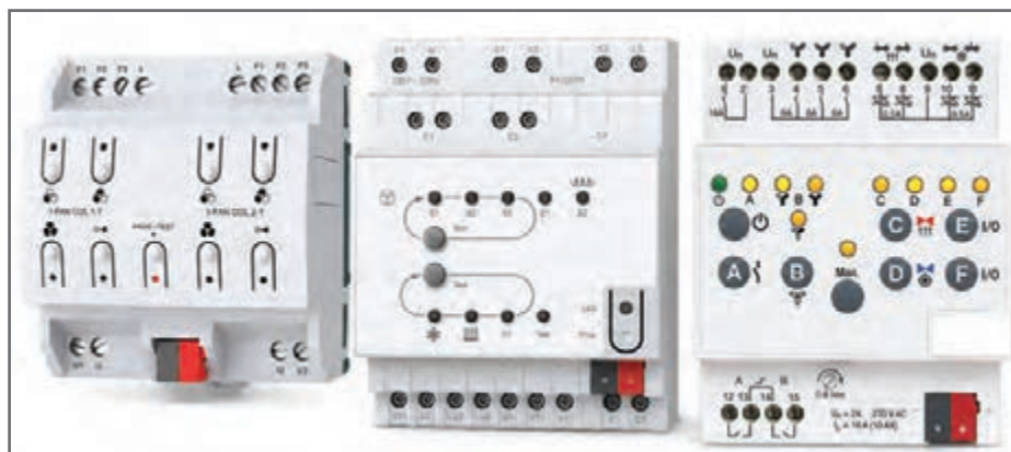
شکل ۲۱- چند نمونه از عملگر سرمایش گرمایش
