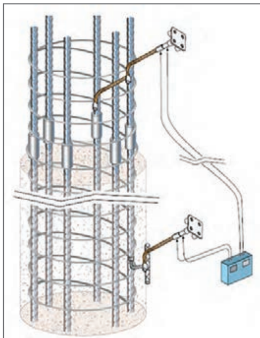
شکل ۲۳- تست مقاومت الکتریکی هم‌بندی
