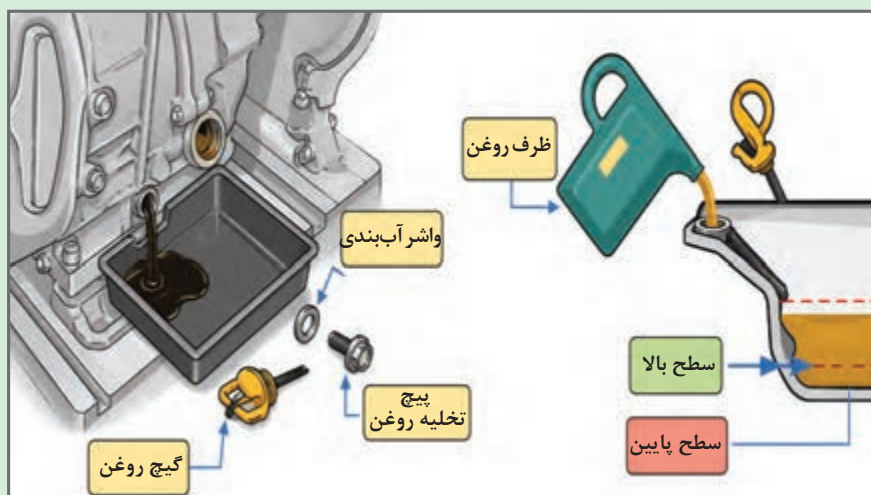
شکل ۳۰- تعویض روغن مولد برق اضطراری
