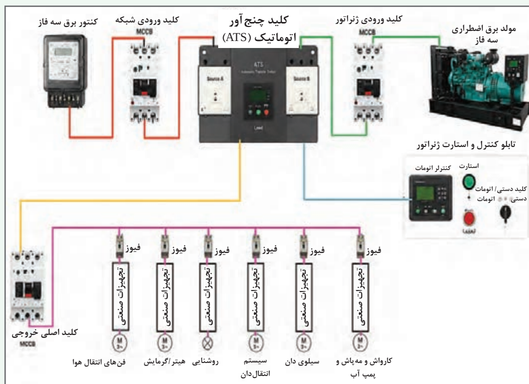
شکل ۲۴- شماتیک تابلو برق مرغداری
