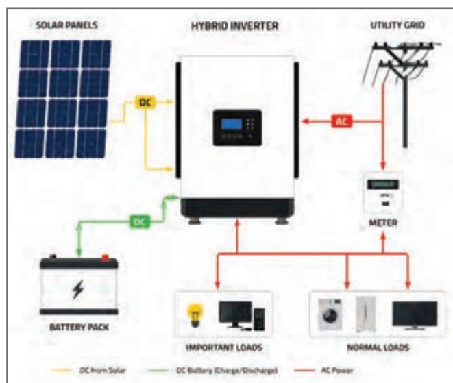
شکل ۳۴- ساختار اتصال اینورتر هیبرید به سیستم فتوولتائیک
