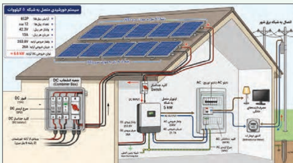
شکل ۴۱- سامانه متصل به شبکه مثال
