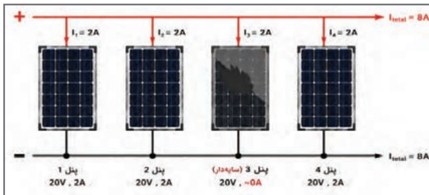
شکل ۲۶- اثر سایه در اتصال موازی
