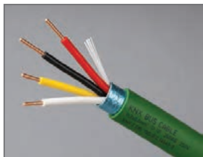
شکل ۱- کابل باس KNX
