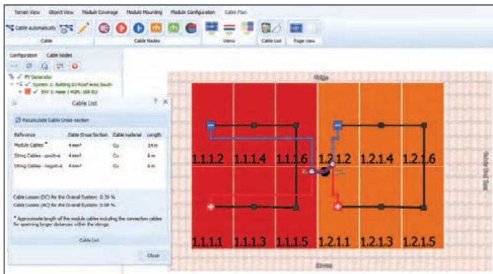
شکل ۵۹- اتصال کابل‌ها
