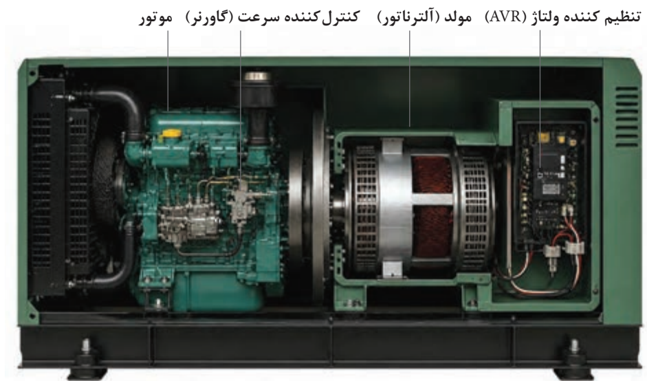
شکل ۲- ساختمان داخلی یک مولد برق اضطراری
