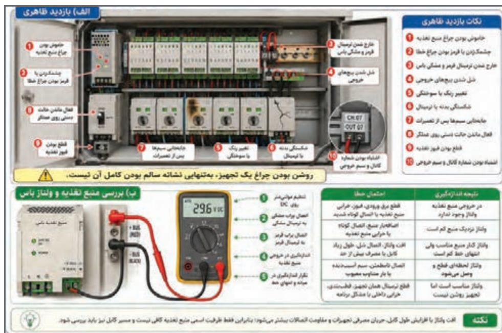
شکل ۴۷- عیب‌یابی شبکه هوشمند
