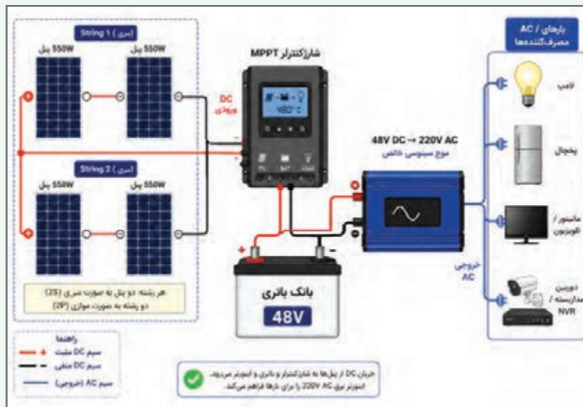
شکل ۷- مدار مثال ۱
