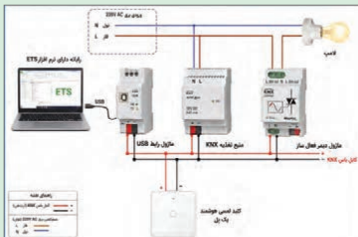
شکل ۲۹- اتصال مدار دایمر
