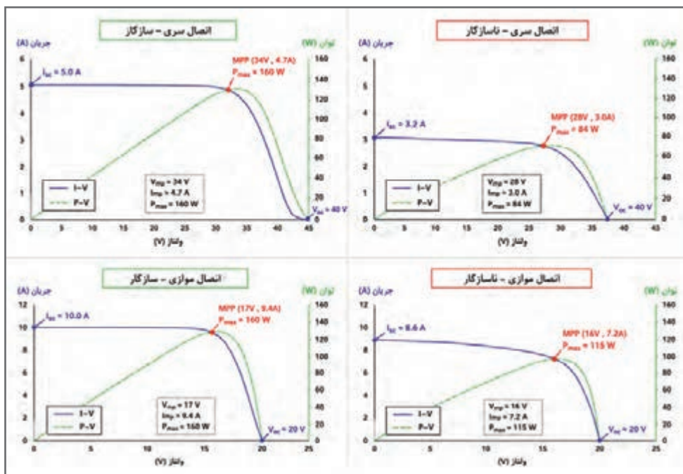
شکل ۳۰- منحنی‌های جریان ولتاژ در دو اتصال سری یا موازی و حالت سازگار و ناسازگار
