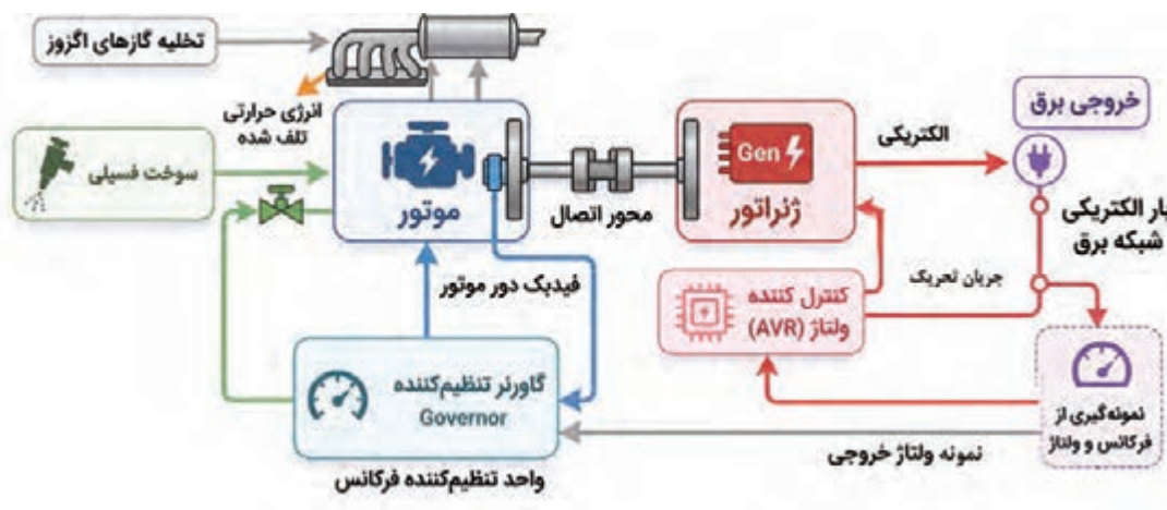
شکل ۵ - هماهنگی اجزای داخلی مولد برق اضطراری
