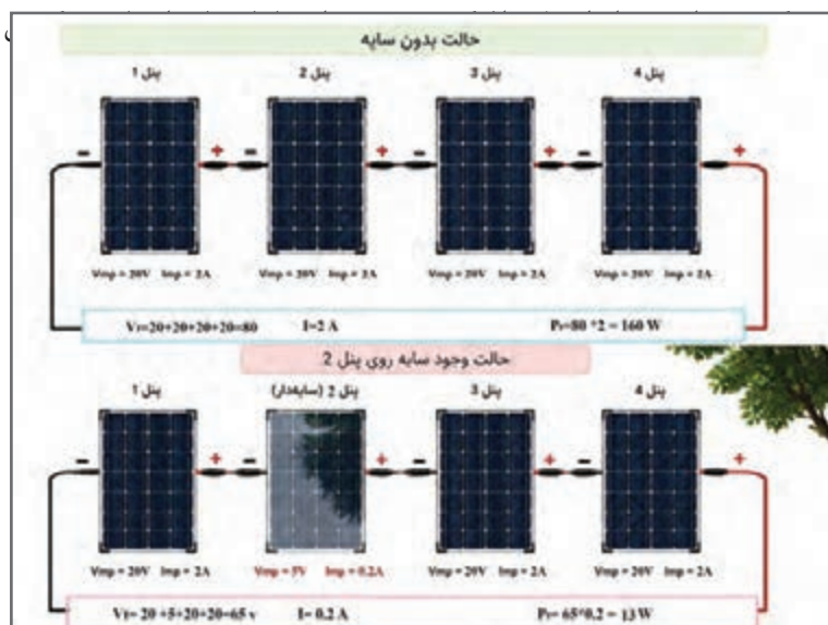
شکل ۲۴- اثر سایه در اتصال سری
