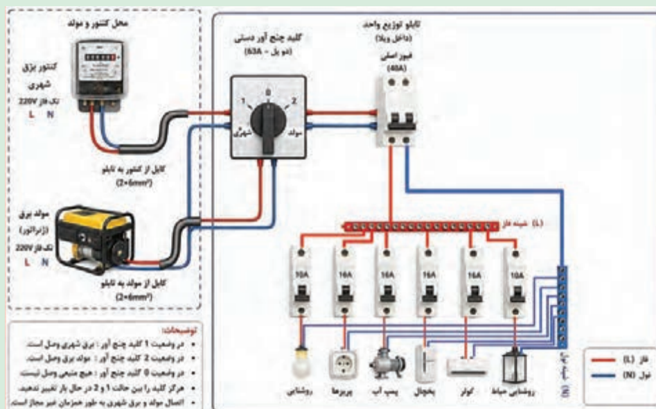
شکل ۲۰- شماتیک تغذیه تابلو برق ویلا با برق شهری و مولد برق (کلید چنج‌آور دستی)
