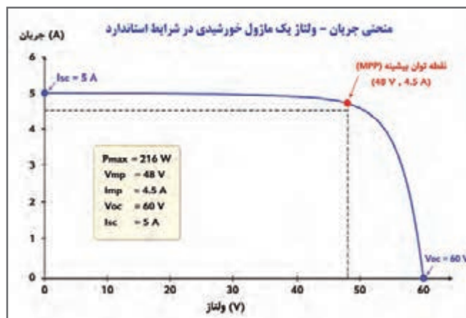
شکل ۲۸- تعیین نقطه کار در منحنی جریان - ولتاژ در شرایط استاندارد
