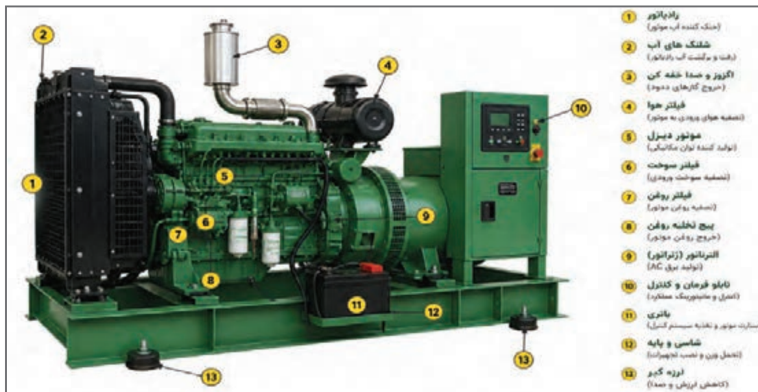
شکل ۱۱- اجزای دیزل ژنراتور
