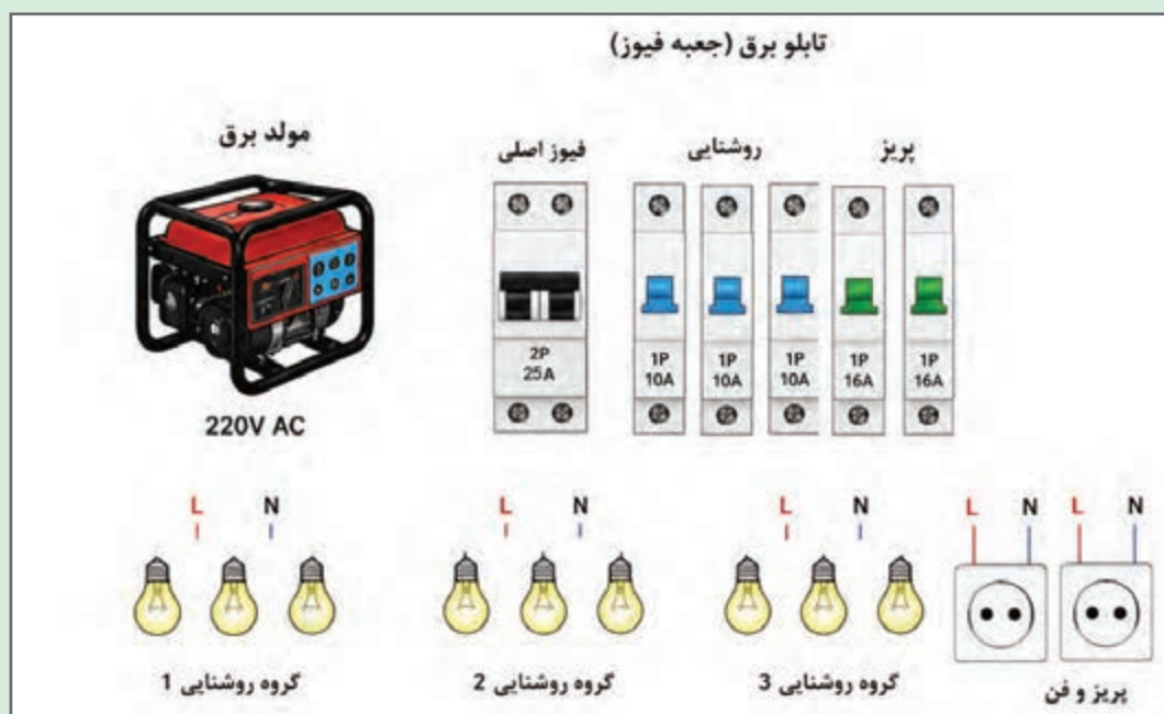
شکل ۱۷- مدار کار عملی
