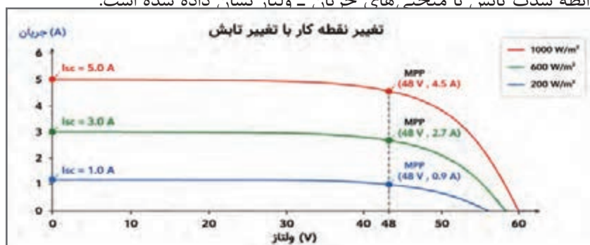
شکل ۲۹- اثر تغییر شدت تابش خورشیدی بر MPP
