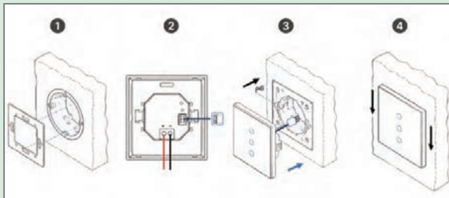
شکل ۷- نصب کلید هوشمند در قوطی
