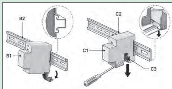
شکل ۶- نصب تجهیزات روی ریل
