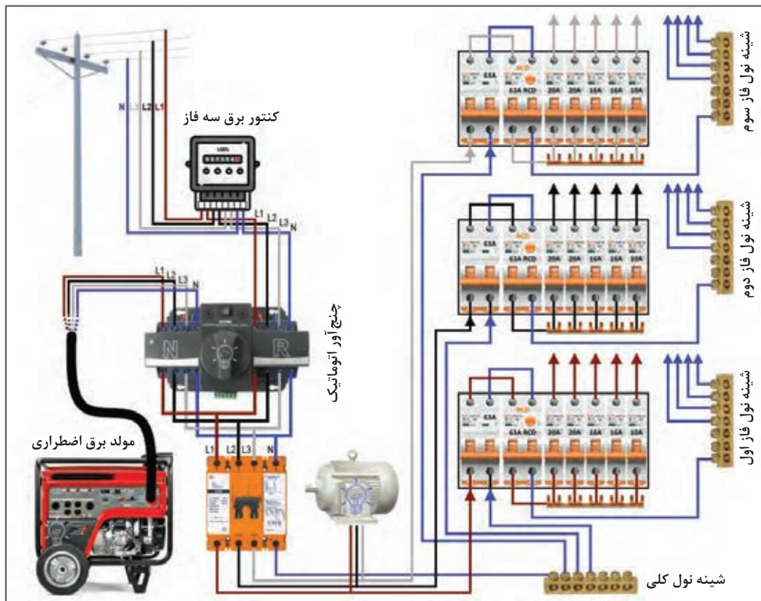
شکل ۲۳ - نحوه اتصال کلید چنج آور اتوماتیک
