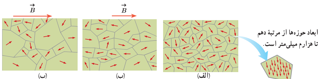
شکل ۳-۲۳ (الف) ماده فرومغناطیسی در نبود میدان مغناطیسی خارجی. (ب) ماده فرومغناطیسی در حضور میدان مغناطیسی خارجی ضعیف. (پ) ماده فرومغناطیسی در حضور میدان مغناطیسی قوی.
