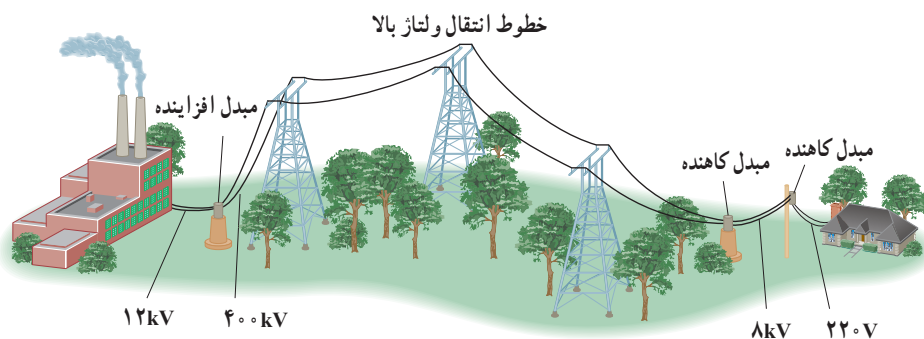
شکل ۳-۳۷ قبل از انتقال توان الکتریکی از نیروگاه ها، مبدل های افزایشده، ولتاژ را تا حدود 400 \text{ kV} افزایش می دهند. در انتهای مسیر، مبدل های کاهنده، ولتاژ را کاهش می دهند تا توان الکتریکی با امنیت بیشتر به محل مصرف برسد.
