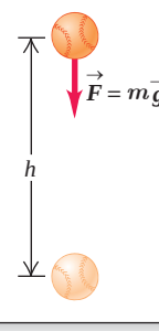
شکل ۱-۲۳ جسم در میدان گرانشی یکنواخت زمین رها می‌شود و به تدریج بر انرژی جنبشی آن افزوده می‌شود.
