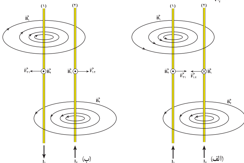
شکل ۳-۱۶ نیروی مغناطیسی‌ای که دو سیم موازی حامل جریان بر یکدیگر وارد می‌کنند.
