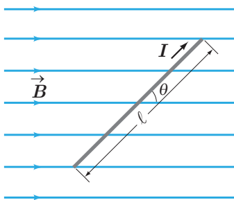
شکل ۳-۱۳ سیم حامل جریان در میدان مغناطیسی.
