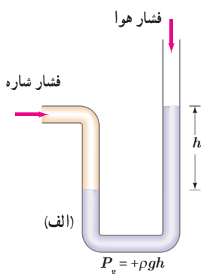
شکل ۱۹-۲ الف) فشار شاره بیشتر از فشار جو است. ب) فشار شاره کمتر از فشار جو است.
