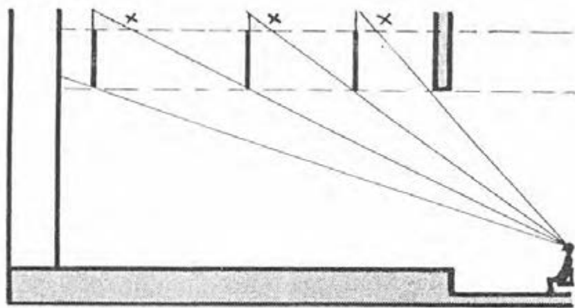
▲ شکل ۵-۸- روش غلط نصب پرده های بالای صحنه که دید تماشاچی را کاملاً کور نمی کند.
