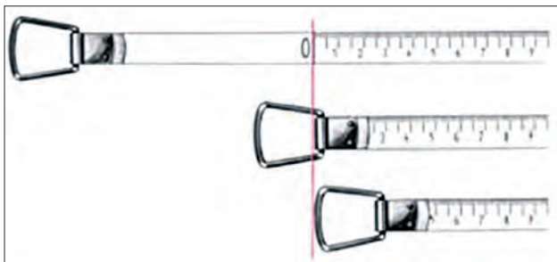
شکل ۲- انواع شروع درجه بندی در نوارهای اندازه گیری
