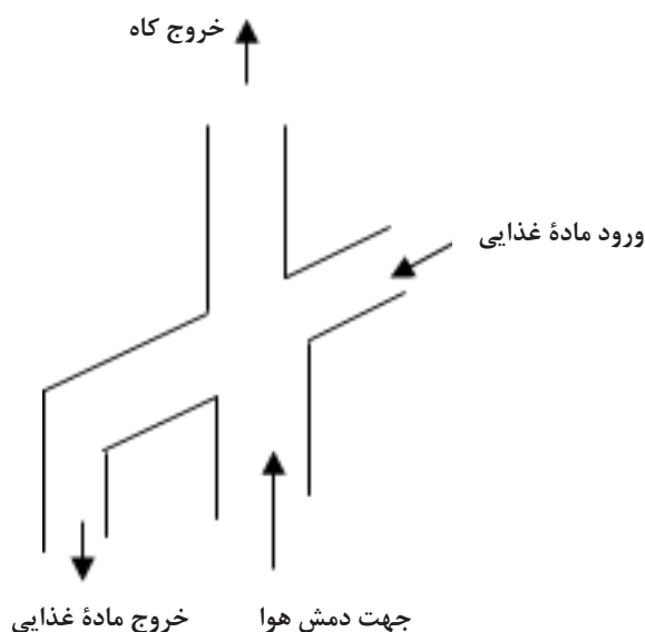
شکل ۱- اصول کار آسپیراتور
