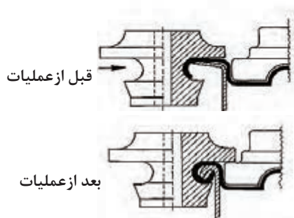
شکل ۷- نحوه عملکرد قرقه های اولیه
