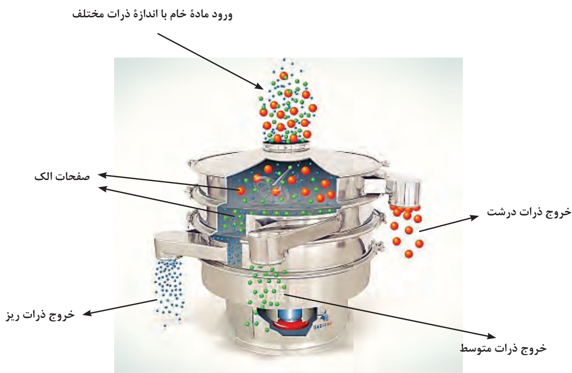
شکل ۸- جداکننده غربالی
