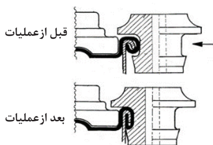
شکل ۸- نحوه عملکرد قرقه های ثانویه
