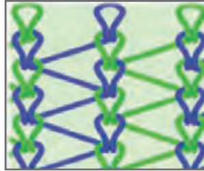
ساختار پارچه حلقوی تاری
