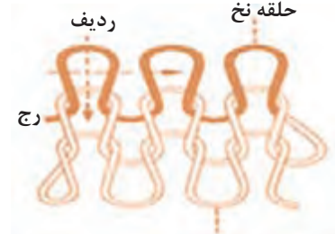
ساختار پارچه حلقوی پودی
