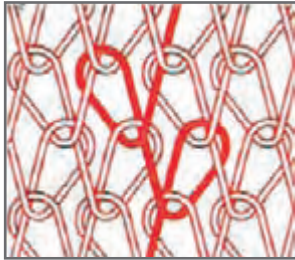
ساختار پارچه حلقوی تاری
