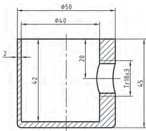
شکل ۴-۲۷- کاسه گردشکن
