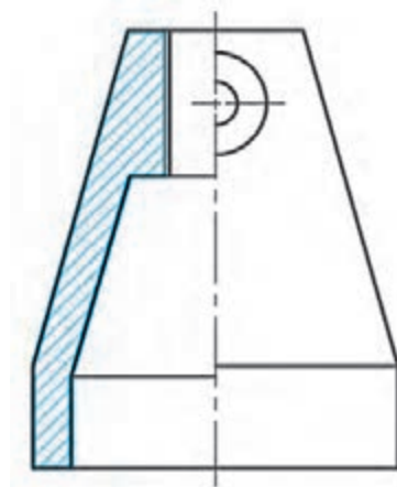
پایه - چدن
