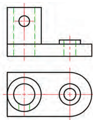
پایه - آلومینیوم
