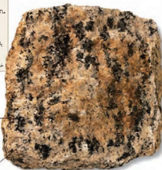
شکل ۲-۲۹- سینیت
