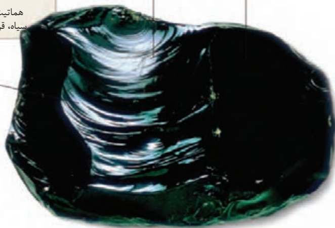
شکل ۲-۲۶- ابسیدین
