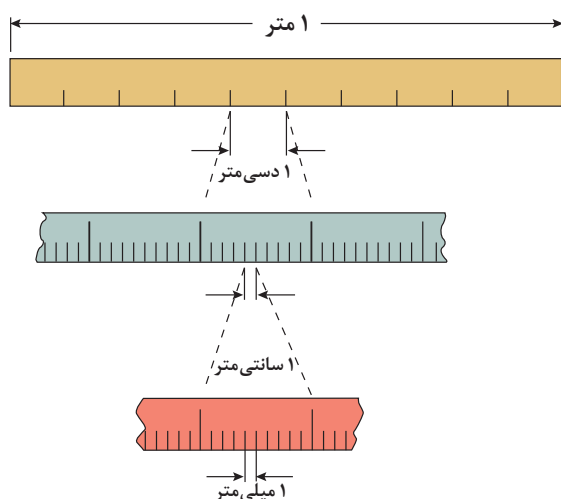
شکل ۷-۱ پیشوندهای کوچک‌کننده یکای متر
