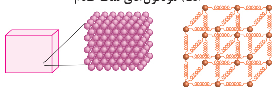
(ب) حرکت ارتعاشی مولکول‌های جامد
