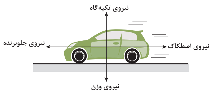
شکل ۱۰-۲ تعادل دینامیکی خودرو
