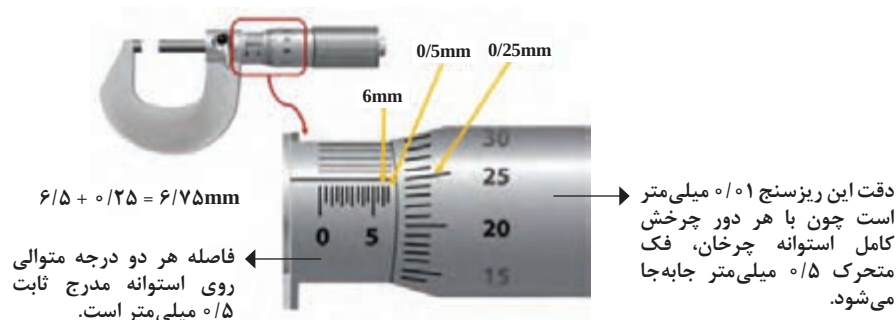
شکل ۱۴-۱ نحوه خواندن نتیجه اندازه‌گیری با ریزسنج ۰/۰۱ میلی‌متری
