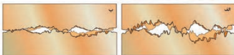
شکل ۲-۲۶ این شکل تأثیر نیروی عمودی تکیه‌گاه بر نیروی اصطکاک را نشان می‌دهد. در شکل الف نیروی عمودی تکیه‌گاه کمتر از شکل ب است و سطح تماس در مقیاس ریز کمتر بوده و نیروی اصطکاک کمتر است.
