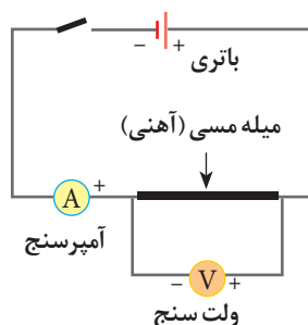
شکل ۱۳-۵ مدار ساده قانون اُهم
