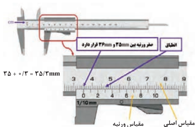
شکل ۱۳-۱ نحوه خواندن نتیجه اندازه‌گیری با کولیس ۰/۱ میلی‌متری
