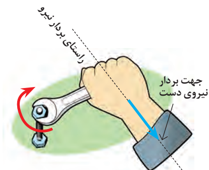
شکل ۱۶-۱ راستا و جهت یک بردار
