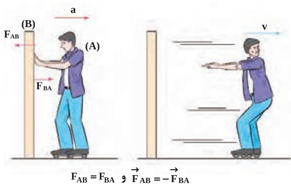
شکل ۲۰-۲ حرکت اسکیت باز به عقب بر اثر نیروی واکنش دیوار
