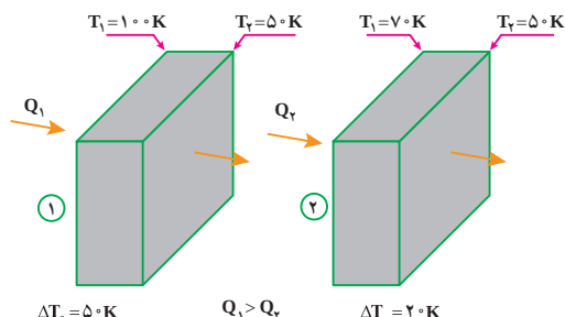
شکل ۴-۸ وابستگی آهنگ رسانش به اختلاف دمای دو سطح
