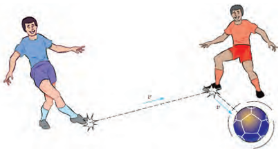
شکل ۱۱-۲ تا زمانی که به جسم نیرویی وارد نشود به حرکت یکنواخت روی خط راست ادامه می‌دهد.
