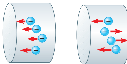
شکل ۳-۵ حرکت الکترون‌های آزاد درون رسانا
