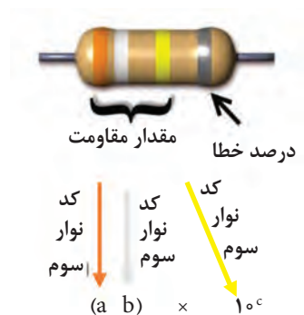
شکل ۵-۱۶ نحوه خواندن مقاومت رنگی
