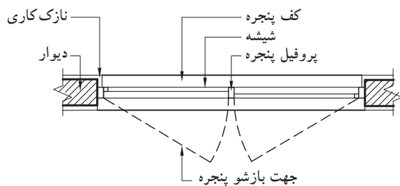
شکل ۱۱۰-۳ پنجره ی دو لنگه ی بازشو
