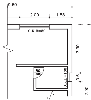
شکل ۱۱۴-۳ طریقه‌ی نوشتن O.K.B در پلان
