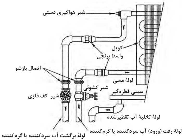
دetailed description of the diagram: This schematic illustrates the piping for a fan coil unit. It shows a coil connected to a water supply and return system. Key components labeled include: شیر هواگیری دستی (Manual air vent valve), کویل (Coil), واسط برنجی (Brass expansion valve), لوله مسی (Copper pipe), اتصال بازشو (Service connection), شیر کف فلزی (Metal floor drain valve), شیر کشویی (Floor drain valve), سینی قطره گیر (Drip tray), لوله تخلیه آب تقطیر شده (Condensate drain pipe), and لوله رفت (ورود) آب سردکننده یا گرم کننده (Supply/return pipe for cooling/heating water). The return pipe is also labeled as لوله برگشت آب سردکننده یا گرم کننده.
