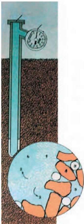
شکل ۱۸-۱- تانسیمتر و نحوه قرار گرفتن آن در خاک
